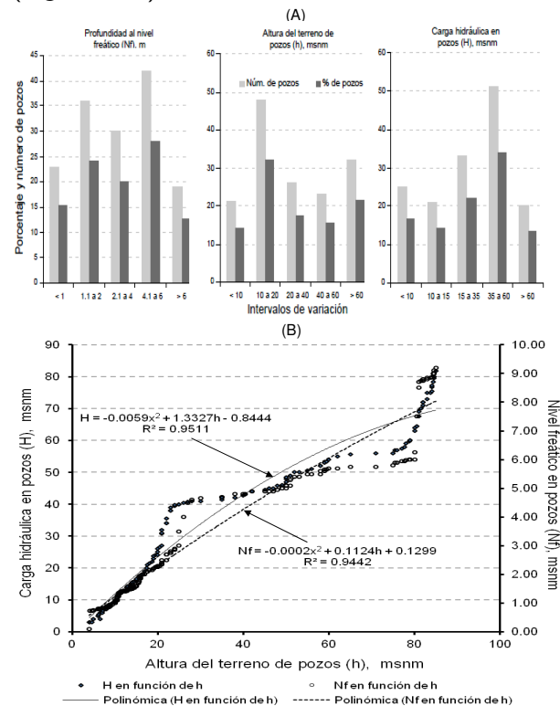
Figura 2. A. Intervalos de valores para el nivel freático (Nf), la altura del terreno (h) y la carga hidráulica (H), según el número y porcentaje de pozos. B. Tendencia y correlación numérica entre H y h, y entre Nf y h, con los respectivos modelos polinómicos (Norzagaray, 2009).
