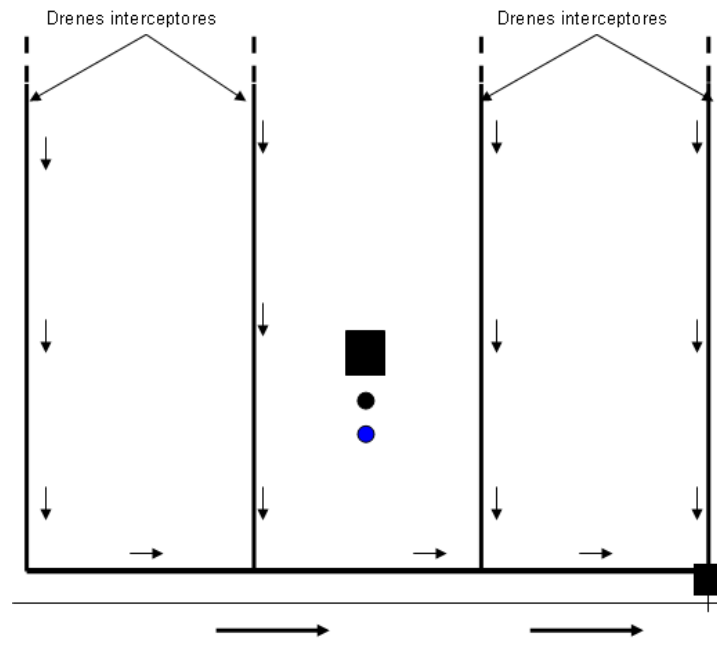
Figura 2. Localización de la zona de muestreo y dispositivos de medición en uno de los espaciamentos de drenaje subterráneo en el lote D-5. ● = pluviómetro, ● = pozo de nivel freático, ■ = zona de muestreo, ■ = estructura de control.
