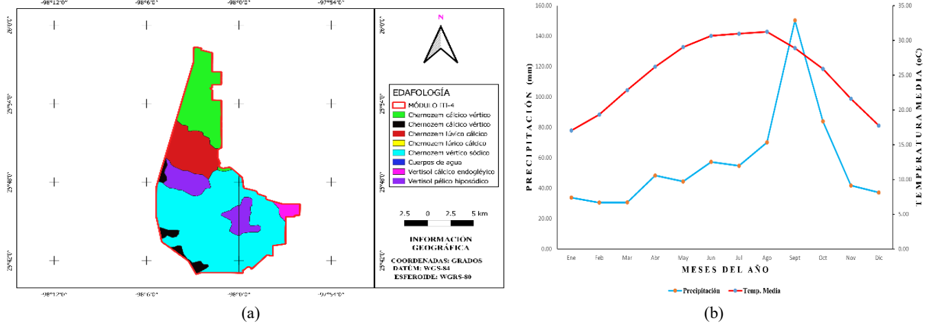
Figura 3. Caracterización edafológica y climática del Módulo III-4: (a) Clasificación de suelos predominantes en el Módulo III-4 según la WRB-2014; (b) Diagrama ombrotérmico relación precipitación y temperatura media anual Módulo III-4. Figure 3. Soil and climatic characterization of Module III-4: (a) Predominant soil classification in Module III-4 based on WRB-2014; (b) Ombrothermic diagram relationship between precipitation and annual mean temperature Module III-4.
