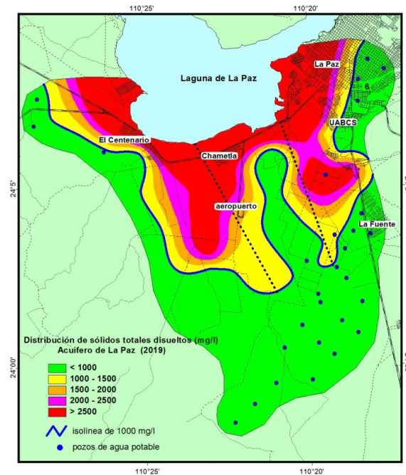
Figura 4. Distribución de STD en el acuífero de La Paz (2019). Se muestran las bandas de concentración de STD, la isolínea de 1000 mg L -1 , y las líneas rectas punteadas donde se midió el desplazamiento anual.
