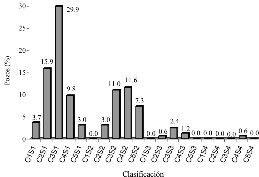
Figura 1. Clasificación del agua del acuífero del Valle del Yaqui, de acuerdo con Richards (1954).
