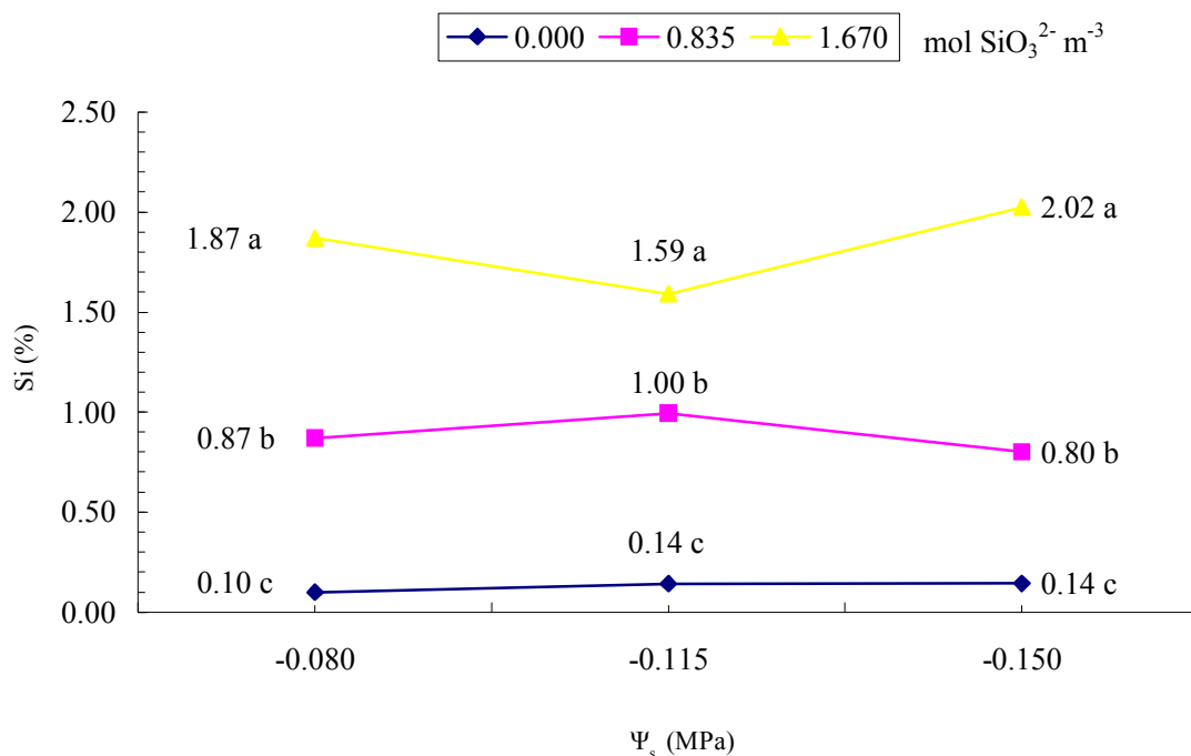
Figura 2. Efecto de potencial osmótico dentro de soluciones nutritivas con diferentes niveles de \text{SiO}_3^{2-} en el contenido de Si de las hojas superiores. Puntos con la misma letra en cada línea son iguales, Scheffe ( P \geq 0.05 ).
