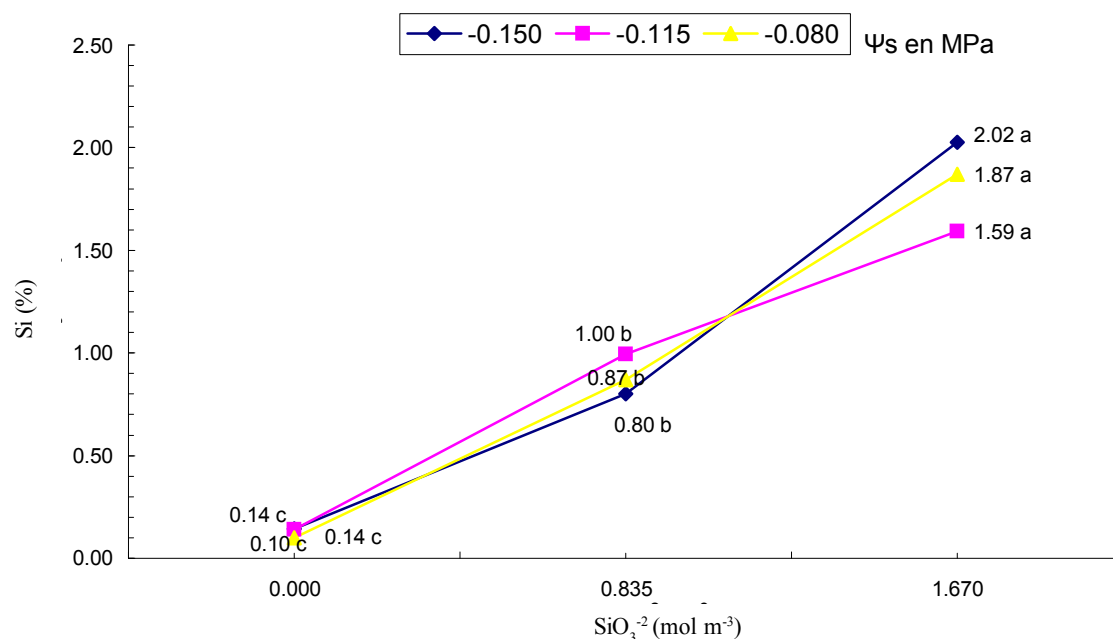
Figura 1. Efecto de silicio dentro de soluciones nutritivas con diferente potencial osmótico en la concentración de Si de las hojas superiores. Puntos con la misma letra en cada línea son iguales, Scheffe ( P \geq 0.05 ).
