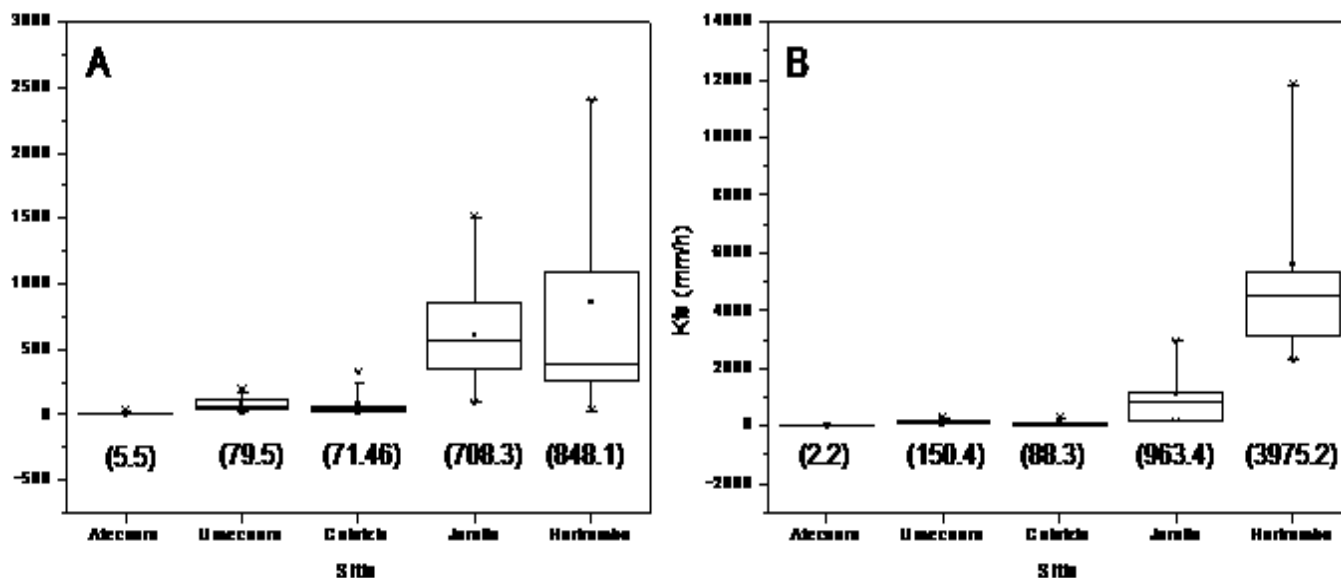
Figura 3. Gráficas de bigotes (desviación estándar) y cajas (error estándar) para la K_{sf} (mm h -1 ) en los diferentes sitios empleando el método Wu1_h1 (A) y Wu2_h1 (B); entre paréntesis se anota el promedio de K_{sf} para cada sitio.
