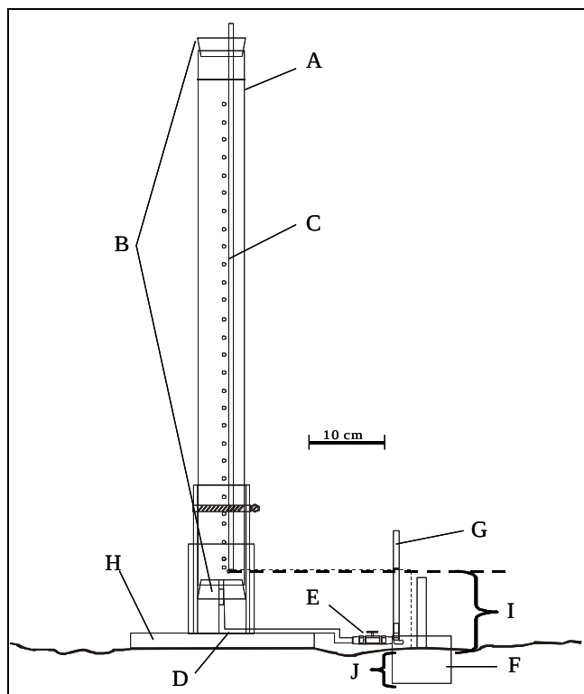
Figura 1. Esquema del IPCCAS armado y montado en campo: A) reservorio principal (Mariotte 63.5 mm diámetro); B) tapones de goma No. 12; C) tubo de burbujeo (9.0 mm diámetro); D) tubo de salida de agua; E) válvula de paso; F) anillo sencillo (88.0 mm diámetro y 80.0 mm longitud); G) tubo de purga y medición de la carga hidráulica (12.0 mm de diámetro por 200.0 mm de longitud); H) base de soporte; I) carga hidráulica constante y J) profundidad de inserción del anillo (60.0 mm).
