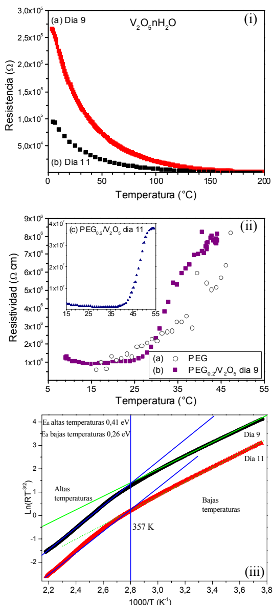
Figura 6. (i) Resistencia eléctrica en función de la temperatura para los precursores V 2 O 5 .nH 2 O para (a) día 9 y (b) día 11 posterior a la reacción. (ii) Resistividad eléctrica en función de la temperatura para (a) el PEG precursor en polvo, (b) las películas PEG/V 2 O 5 , obtenidas los días 9 y (c) 11 posterior a la reacción. (iii).
