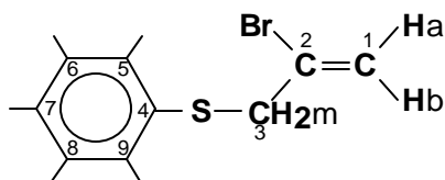
Fig. 1. Descripción del sistema magnético para el fragmento -\text{CH}_2\text{CBr}=\text{CH}_2 y numeración de los átomos de carbono.
