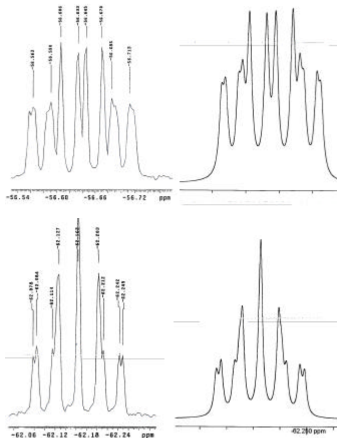
Fig. 2. Espectros de RMN ^{19}\text{F} , experimentales (izq.) y simulados (der.), para el sistema \text{AA}'\text{BB}'\text{X} en el compuesto \text{C}_6\text{HF}_4\text{-2,3,5,6-SCH}_2\text{CBrCH}_2 2 .
