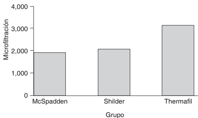
Figura 3. Microfiltración apical de las tres técnicas de obturación.
