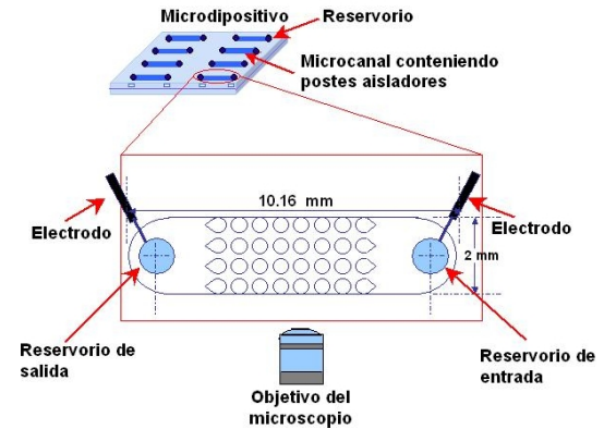
Fig. 2. Representación del microdispositivo y de un microcanal con los obstáculos aisladores.
