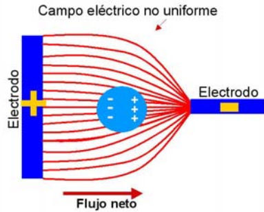
Fig. 1. Movimiento de una partícula en un campo eléctrico no uniforme (dielectroforesis positiva).
