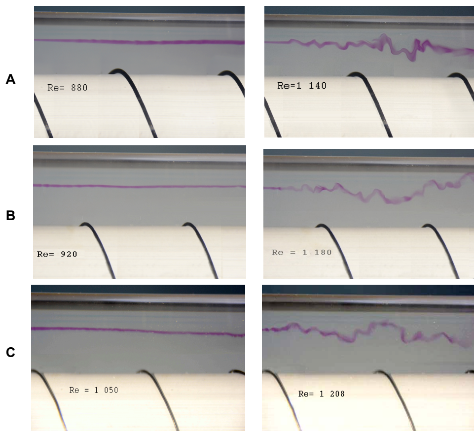
Fig. 6. Fotografías tomadas para identificar el cambio en la hidrodinámica del flujo en espacios anulares rectos con espirales insertadas a partir de la inyección de tinta. A - Espiral ( e = 1.5 mm). B - Espiral ( e = 1.0 mm). C - Espiral ( e = 0.5 mm).
