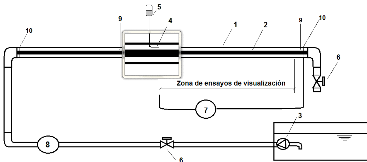
Fig. 1. Esquema de la instalación con los elementos que la componen. (1) Tubo exterior deacrílico. (2) Tubo interior de cobre. (3) Bomba sumergible. (4) Aguja inyectora. (5) Depósito de tinta. (6) Válvulas. (7) Manómetro diferencial. (8) Flujómetro de Coriolis. (9) Termómetros. (10) Elementos de soporte.
