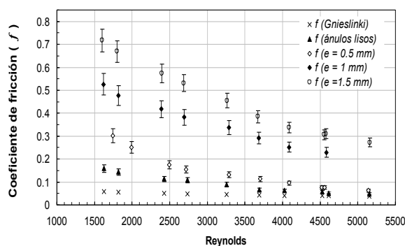
Fig. 8. Factor de fricción para el flujo en ánuos lisos y con la incorporación de las espirales de diámetro de hilo ( e ) de: 0.5 mm, 1 mm y 1.5 mm.
