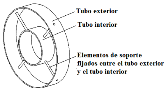
Fig. 2. Representación de los elementos de soporte usados para mantener concéntrico el tubo interno en el ánulo.
