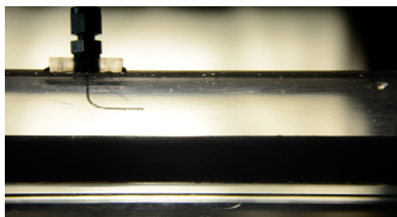
Fig. 3. Detalle de la inyección de tinta en el espacio anular.
