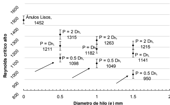
Fig. 7. Valores para el número de Reynolds crítico para las espirales insertadas en el espacio anular.
