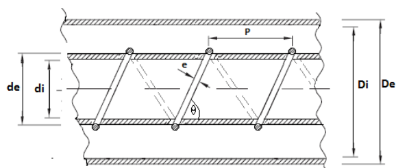
Fig. 4. Espirales helicoidales insertadas en un espacio anular y las geometrías que caracterizan esta inserción.
