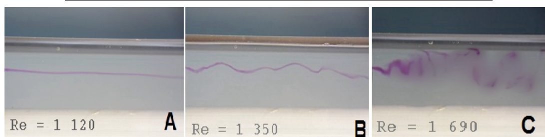
Fig. 5. Fotografías tomadas para identificar la hidrodinámica en espacios anulares rectos y lisos a partir de la inyección de tinta. A - Flujo laminar estable. B - Flujo laminar ondulado con ligeras oscilaciones del flujo. C- Flujo turbulento establecido.
