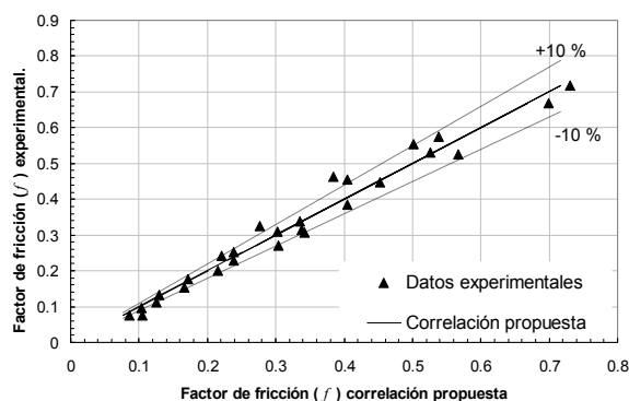
Fig. 9. Comparación entre el coeficiente de fricción obtenido experimentalmente y el predicho por la Ec. (8) propuesta.
