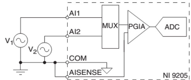
Figura 6: Diagrama de conexión del NI-9205 en configuración NRSE.
