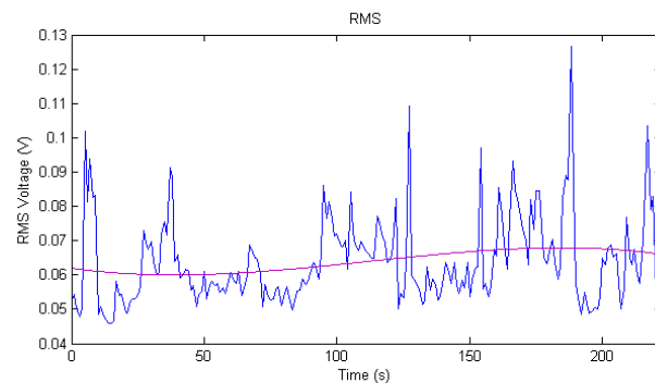
Figura 13: Voltaje RMS de la señal SEMG obtenida.
