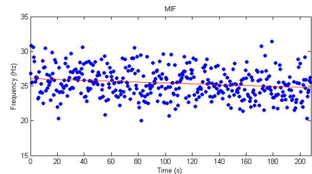
Figura 15: IMNF junto con su recta de tendencia lineal para contracciones dinámicas.
