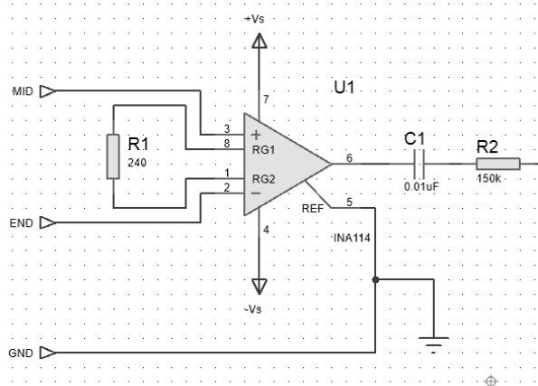
Figura 2: Circuito de la etapa de amplificación.
