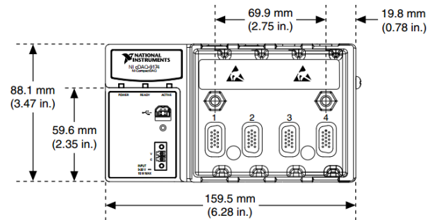
Figura 5: Chasis NI cDAQ USB de 4 Ranuras.
