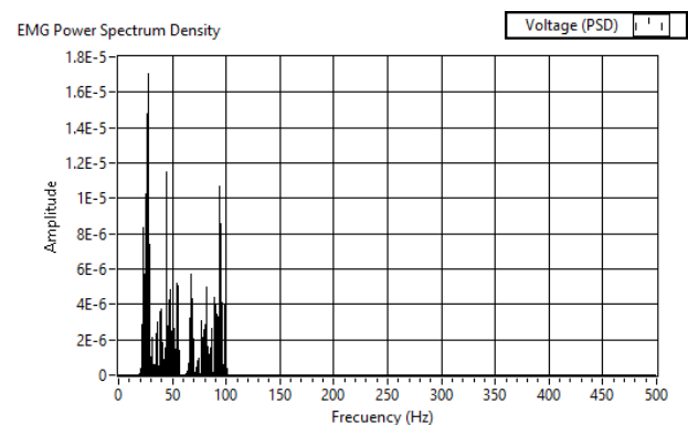
Figura 11: PSD de la señal EMG durante un instante de tiempo.
