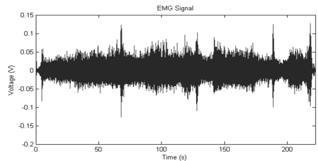
Figura 10: Señal SEMG obtenida durante una contracción estática.
