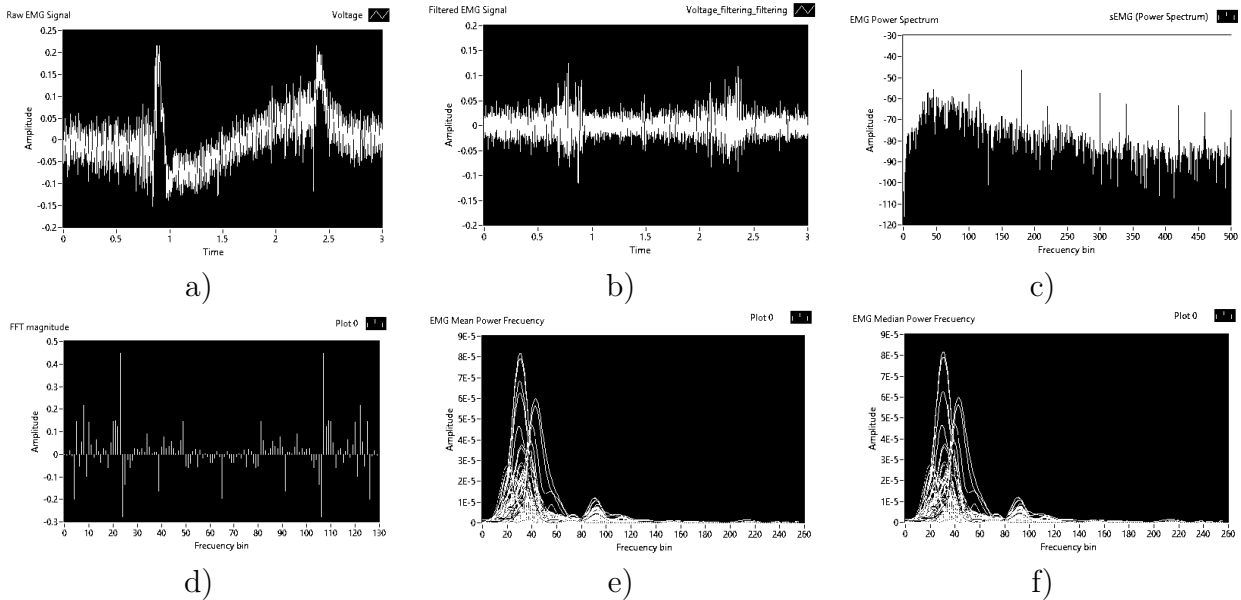
Figura 9: Sistema de procesamiento de señales digitales. Señal SEMG en bruto (a), Señal SEMG después del filtrado digital (b), Espectro de potencia de la señal (c), Magnitud de la FFT (d), Frecuencia de potencia mediana (e), Frecuencia de potencia media (f).
