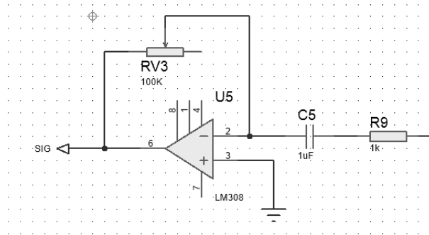
Figura 4: Circuito filtro pasa altas.
