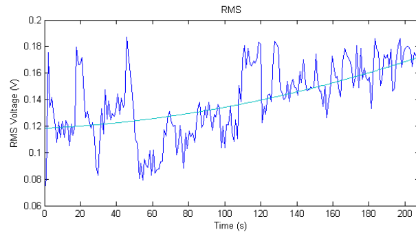
Figura 16: Voltaje RMS de la señal SEMG obtenida de contracciones dinámicas.
