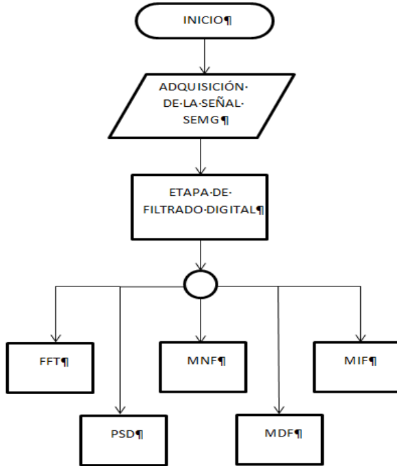
Figura 7: Diagrama de flujo del software.
