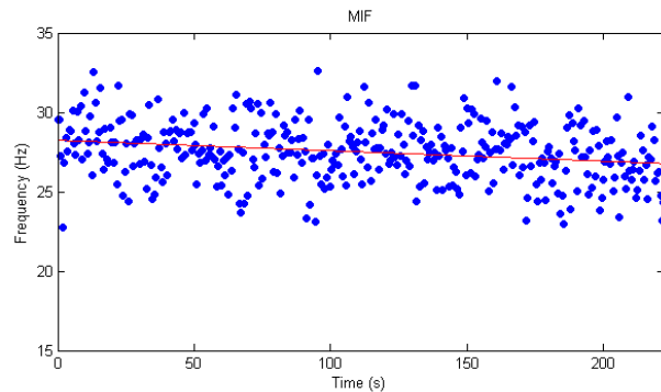
Figura 12: IMNF junto con su recta de tendencia lineal.
