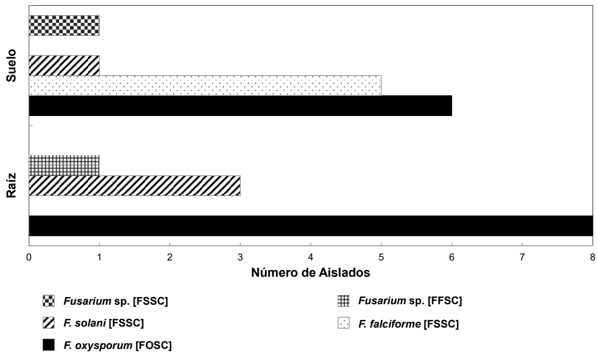
Figura 4. Frecuencia de especies/complejo en 25 cepas de Fusarium spp. seleccionadas de un acervo de 109 cepas aisladas de suelo y raíz en cuatro condiciones fitosanitarias y previamente caracterizadas morfológica y culturalmente. Verano, 2016. Los Altos, Jalisco.
