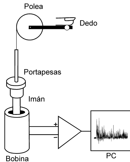
FIGURA 1. Esquema del dispositivo utilizado para medir el movimiento lento del dedo índice. Se ha agregado a este dispositivo un potenciómetro polarizado cuyo eje está alineado con el eje de la polea.
