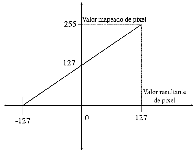
FIGURA 2. Ajuste de los valores de píxel por medio de una transformación lineal. De esta manera se evitan los valores negativos en el píxel resultante en las componentes C1 , C2 , y C3 .
