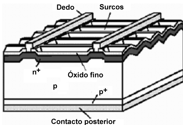
FIGURA 4. Estructura de celda solar con emisor selectivo.
