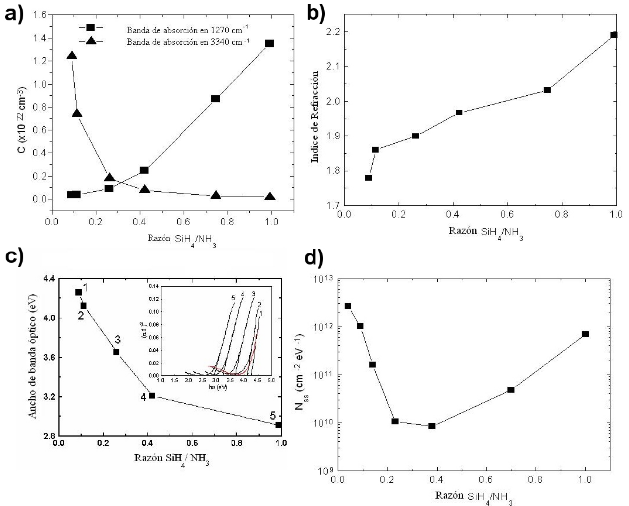
FIGURA 8. Diversas propiedades de las capas de SiN:H obtenidas por PECVD en función de la relación de presiones parciales de \text{SiH}_4/\text{NH}_3 . (A) Concentración de enlaces Si-H y N-H; (B) Índice de refracción; (C) Ancho de banda prohibida y (D) densidad de estados a la mitad de banda prohibida en la superficie del silicio.
