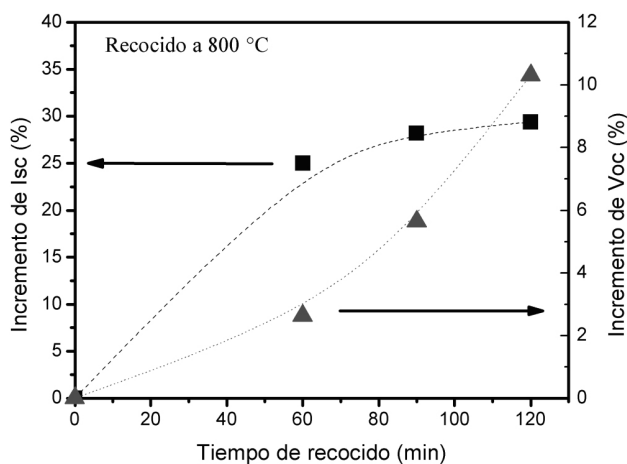
FIGURA 12. Incrementos relativos de J_{sc} y V_{oc} en función del recocido a 800^{\circ}\text{C} en gas forming .
