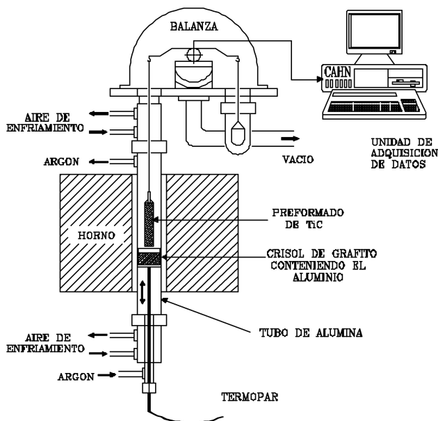
FIGURA 1. Sistema experimental empleado para realizar la infiltración.
