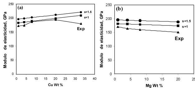
FIGURA 5. Modulo de elasticidad de los materiales compuestos, (a) en función del contenido de Cu y (b) en función del contenido de Mg.
