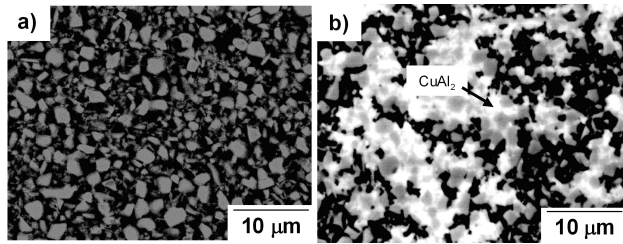
FIGURA 3. Microestructura de los materiales compuestos infiltrados a 900°C. (a) Al-20Mg/TiC y (b) Al-20Cu/TiC.
