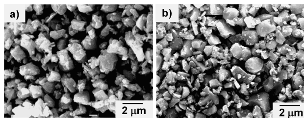
FIGURA 2. (a) Morfología de los polvos de TiC; (b) microestructura de los preformados sinterizados parcialmente a 1250^\circ\text{C} .
