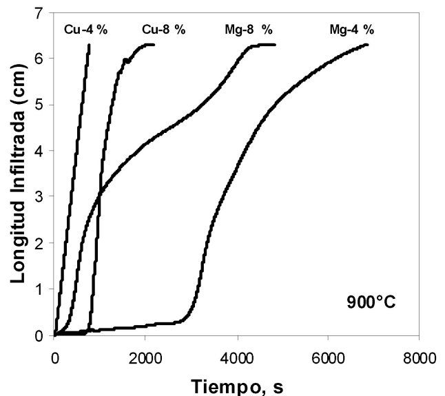
FIGURA 7. Comparación de la velocidad de infiltración de los materiales compuestos \text{AlCu}_x/\text{TiC} y \text{AlMg}_x/\text{TiC} a 900^\circ\text{C} .
