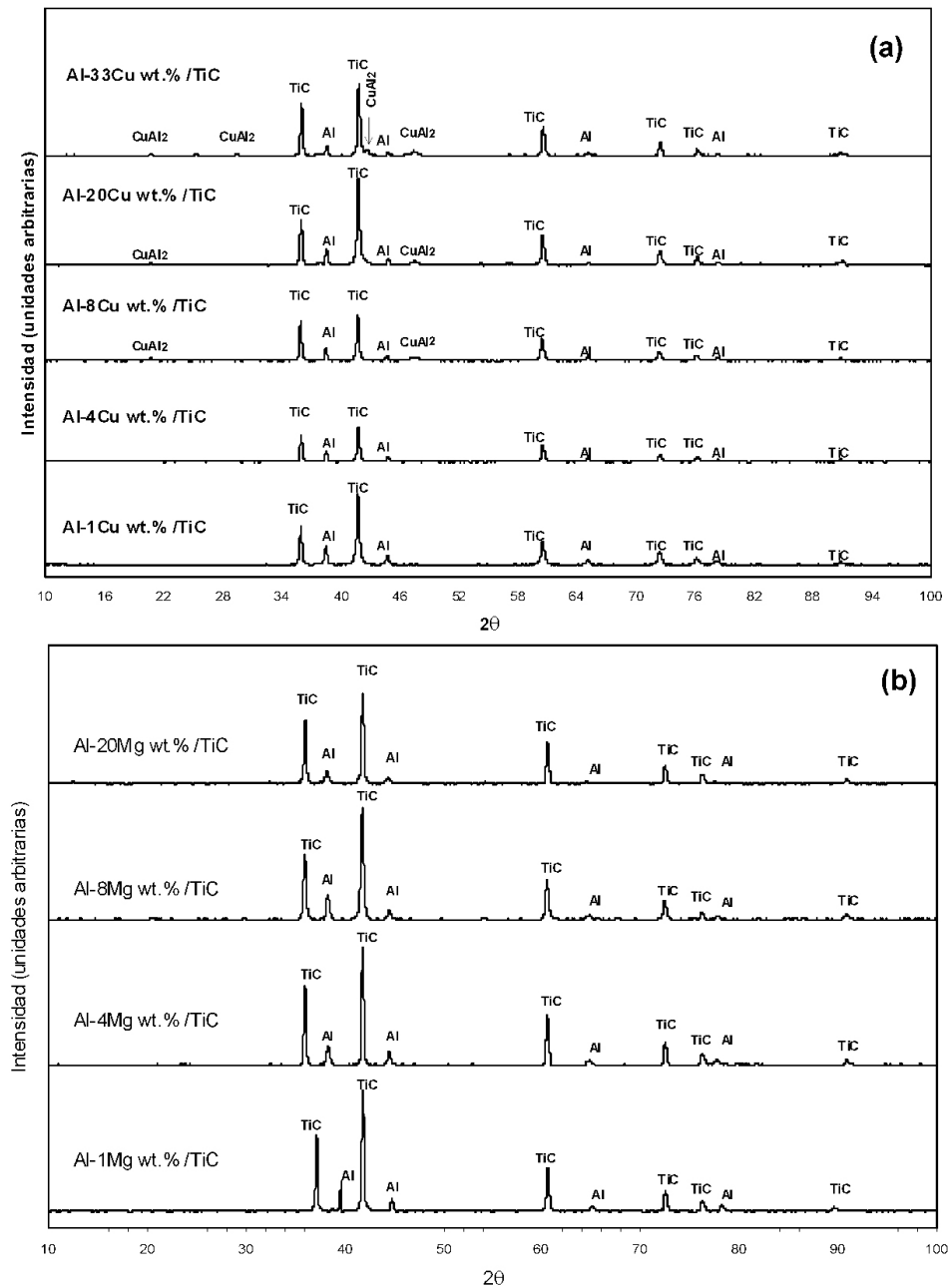
FIGURA 4. Espectros obtenidos por difracción de rayos X de los materiales compuestos. (a) AlCu x /TiC y (b) AlMg x /TiC.
