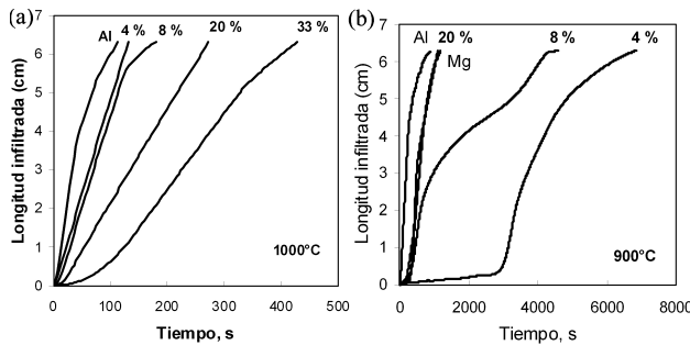
FIGURA 6. Curvas de infiltración de los materiales compuestos (a) Compuestos \text{AlCu}_x/\text{TiC} infiltrados a 1000^\circ\text{C} , (b) Compuestos \text{AlMg}_x/\text{TiC} infiltrados a 900^\circ\text{C} .
