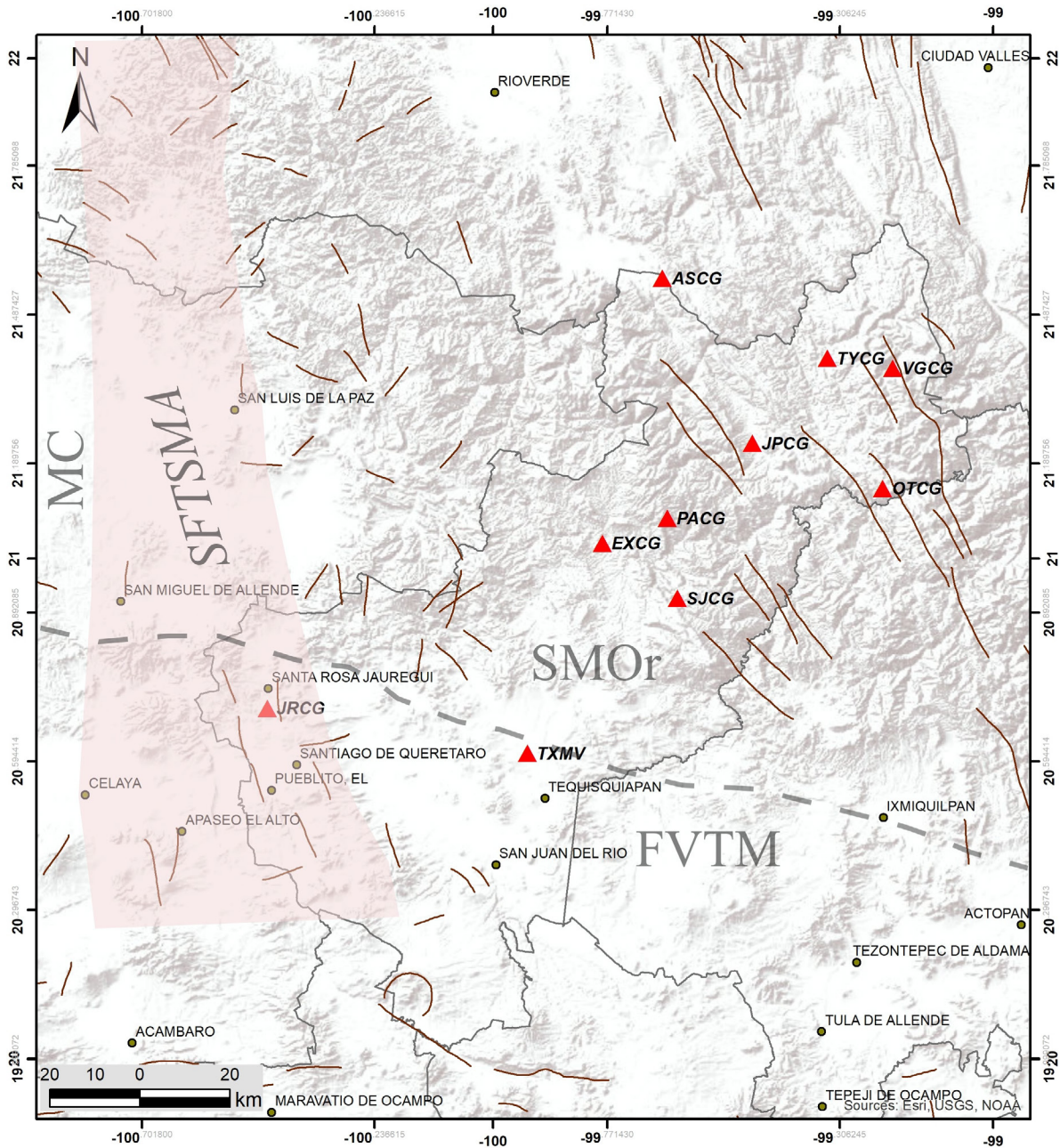
Figura 3. Provincias fisiográficas en el estado de Querétaro. SMOr: Sierra Madre Oriental, FVTM: Faja Volcánica Transmexicana, MC: Mesa Central, SFTSMA: Sistema de Fallas Taxco San Miguel de Allende. Las líneas café indican las fallas en la región y los triángulos la ubicación de las estaciones de la Red Sísmica de Querétaro.
