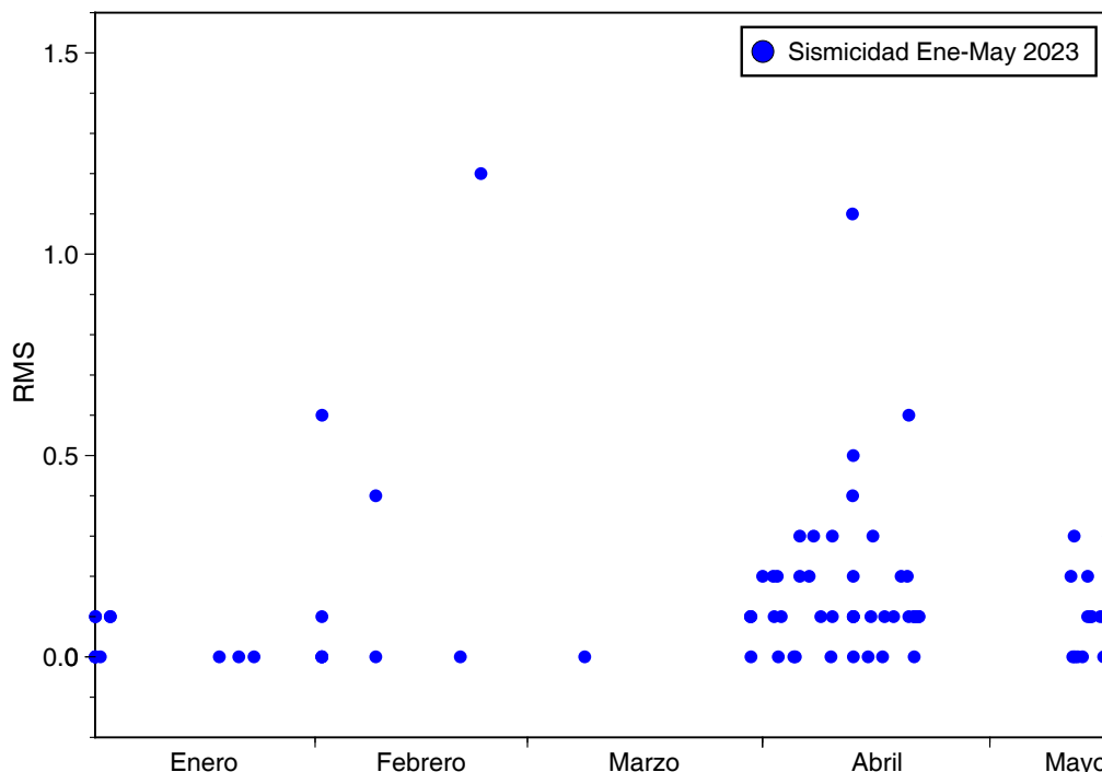
Figura 8. Error RMS para la sismicidad mostrada en la Figura 7. El aparente incremento de sismicidad, de izquierda a derecha, se debe a la mejora en el algoritmo de disparo basado en la relación STA/LTA. El RMS se incrementa conforme los epicentros ocurren más lejos de la red, lo mismo ocurre con algunos eventos en los que la relación señal-ruido disminuye.
