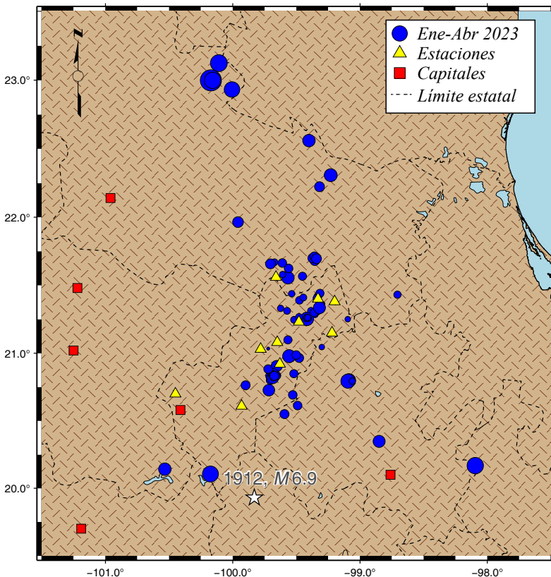
Figura 7. Microsismicidad registrada por la ReSiQ (círculos azules) de enero a mediados de mayo de 2023. Los epicentros en la Sierra Gorda conservan la misma tendencia de los eventos de la Figura 5. Nótese una concentración de eventos antropogénicos, con dirección SW-NE, en la parte centro este del estado de Querétaro, entre las estaciones SJCJ y TXMV.
