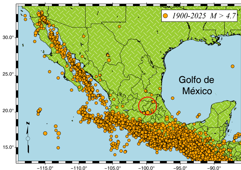
Figura 1. Ubicación de la región de estudio (círculo rojo). Sismicidad registrada por el SSN de enero de 1900 a febrero de 2025 ( 4.7 < M < 8.2 ).
