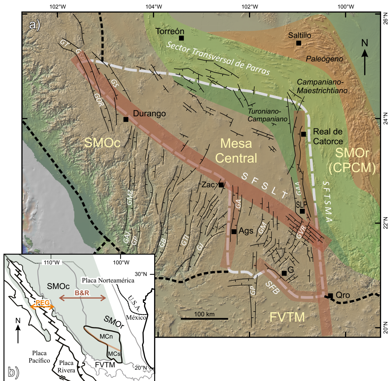
Figura 1. Escenario tectónico y fisiografía de la región central y norte de México. En el modelo digital de elevación (obtenido de GeoMapApp - http://www.geomapp.org/ ) se muestra la localización de las estructuras mayores de la Mesa Central y las zonas aledañas. El sistema de fallas San Luis-Tepehuanes (SFSLT) divide a la MC en dos partes, norte y sur. Las franjas coloreadas de la parte superior derecha indican la temporalidad de las estructuras de acortamiento del Cinturón de Pliegues y Cabalgaduras Mexicano de acuerdo con Fitz-Díaz et al. (2018). GA: Graben de Aguascalientes; GAA: Graben Arista-Ahualulco; GAJ: Graben Álica-Jesús María; GB: Graben Bolaños; GJ: Graben de Juchipila; GM: Semigraben de Matancillas; GMZ: Graben Mezquital; GOR: Graben Otinapa-Río Chico; GP: Graben Pajaritos; GPP: Graben Penjamillo-Pinos; GS: Graben de Santiaguillo; GSP: Semigraben de Santiago Papasquiaro; GT: Graben de Tepehuanes; GTL: Graben de Tlaltenango; GVR: Graben de Villa de Reyes; SFB: Sistema de Fallas del Bajío; SFTSMA: Sistema de Fallas Taxco-San Miguel de Allende. B&R: Provincia Basin and Range meridional; CPCM: Cinturón de Pliegues y Cabalgaduras Mexicano; FVTM: Faja Volcánica Transmexicana; MC: Mesa Central; MCn Mesa Central parte norte; MCs: Mesa Central parte sur; PEG: Provincia Extensional del Golfo; SMOc: Sierra Madre Occidental; SMOr: Sierra Madre Oriental. Ags: Aguascalientes; G: Guanajuato; Qro: Querétaro; SLP: San Luis Potosí; Zac: Zacatecas
