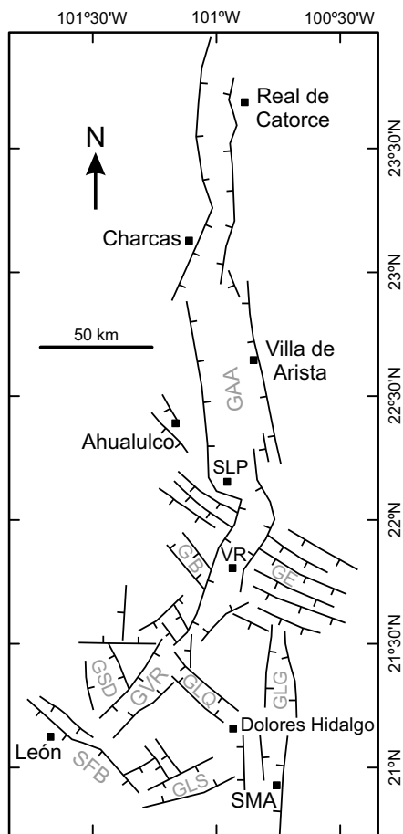
Figura 9. Esquema estructural del graben de Villa de Reyes. GB: Graben de Bledos; GAA: Graben Arista-Ahualulco; GLG: Graben La Granja; GLQ: Graben La Quemada; GLS: Graben de La Saucedá; GSD: Graben Santo Domingo; GVR: Graben de Villa de Reyes; SFB: Sistema de Fallas del Bajío. SLP: San Luis Potosí; SMA: San Miguel de Allende; VR: Villa de Reyes.
