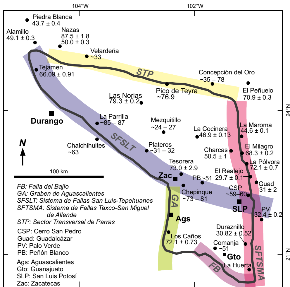
Figura 3. Esquema de la Mesa Central mostrando la localización de intrusivos y sus edades. Los números son las edades (Ma) con su respectivo error ( \pm 2\sigma ). Los trabajos de donde se obtuvieron las edades y otra información complementaria son presentados en la Tabla 1.
