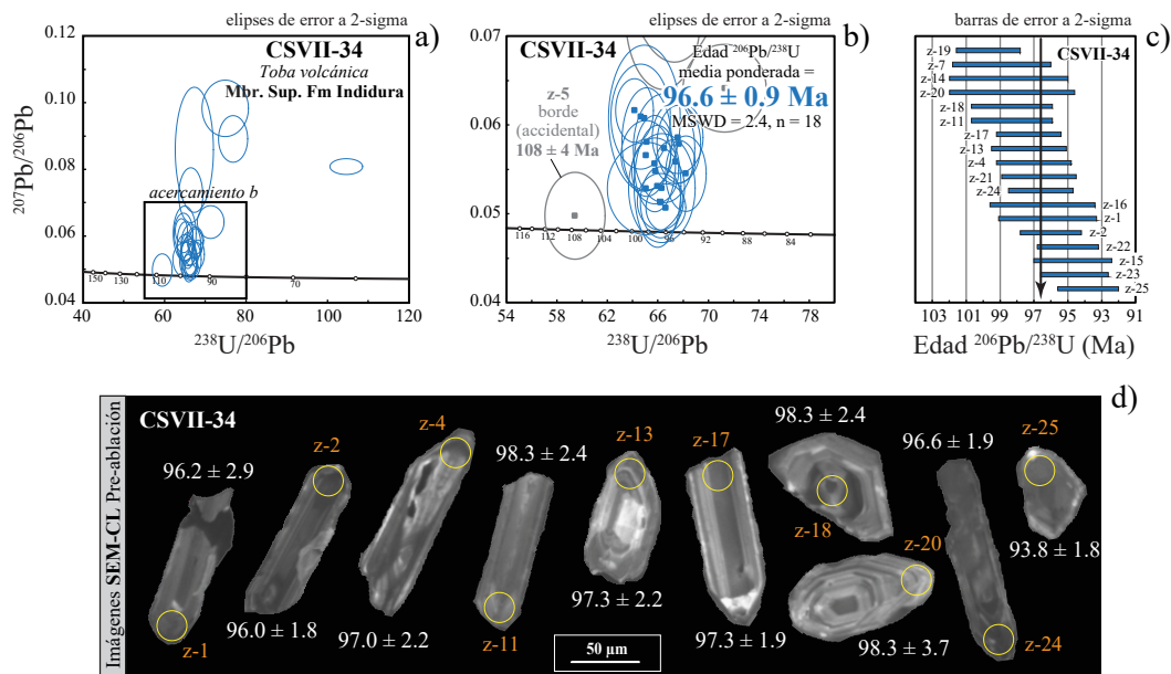
Figura 7. Edades U-Pb en la muestra clave CSVII-34. a) Gráfico de concordia tipo Tera Wasserburg mostrando todos los datos de los granos de circón analizados; b) esta imagen corresponde a un acercamiento del gráfico a, en ella también se muestra la edad ^{206}\text{Pb}/^{238}\text{U} media ponderada de 96.6 \pm 0.9 Ma. Se observa en color gris un grano de circón con edad discordante; c) gráfico de las edades de granos de circón utilizados para calcular la media ponderada; d) imágenes de catodoluminiscencia de granos de circón representativos de la muestra obtenidos por SEM.
