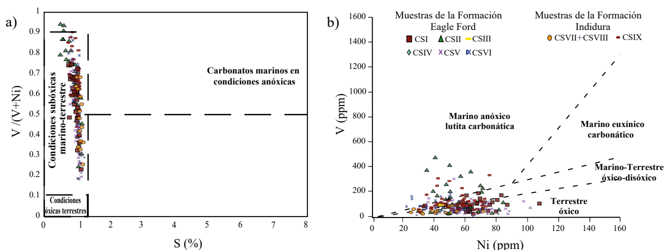
Figura 12. a) Gráfico de las proporciones de elementos traza de V/(V+Ni) versus el contenido de azufre en porcentaje ( S %), que muestra que las condiciones de deposición de las rocas generadoras son similares y que se depositaron en condiciones subóxicas marino-terrestres (Lewan, 1984. Gráfico tomado de Al-Khafaji et al. , 2020). b) Zonación gráfica de las concentraciones de vanadio ( V ) y níquel ( Ni ) para interpretaciones paleoambientales (Galarraga et al. , 2008), que muestra variaciones entre condiciones óxicas, óxido-disóxicas y anóxicas de las Formaciones Eagle Ford e Indidura, donde las columnas CSII, CSV, CSVI, CSIX caen en condiciones mayormente marino-anóxicas.
