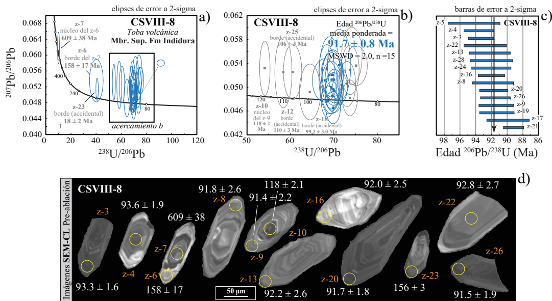
Figura 10. Edades U-Pb en la muestra clave CSVIII-8. a) Gráfico de concordia tipo Tera Wasserburg mostrando todos los datos de los granos de circonio analizados; b) esta imagen corresponde a un acercamiento del gráfico A, en ella también se muestra la edad ^{206}\text{Pb}/^{238}\text{U} media ponderada de 91.7 \pm 0.8 Ma. Las elipses de color gris representan herencias de granos de circonio, plomo común y/o pérdida de plomo; c) gráfico de las edades de granos de circonio utilizados para calcular la media ponderada; d) imágenes de catodoluminiscencia de granos de circonio representativos de la muestra obtenidos por SEM.
