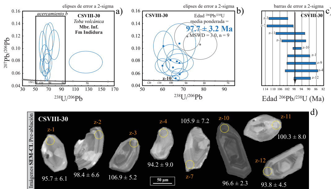
Figura 8. Edades U-Pb en la muestra clave CSVIII-30. a) Gráfico de concordia tipo Tera Wasserburg mostrando todos los datos de los granos de circón analizados; b) esta imagen corresponde a un acercamiento del gráfico a, en ella también se muestra la edad ^{206}\text{Pb}/^{238}\text{U} media ponderada de 97.7 \pm 3.2 Ma. Las elipses de color azul son las que fueron empleadas para calcular la edad media ponderada, mientras que las elipses de color gris fueron descartadas para el cálculo de esta edad, debido a que representan granos de circón más discordantes, plomo común y/o pérdida de plomo; c) gráfico de las edades de granos de circón utilizados para calcular la media ponderada; d) imágenes de catodoluminiscencia de granos de circón representativos de la muestra obtenidos por SEM.
