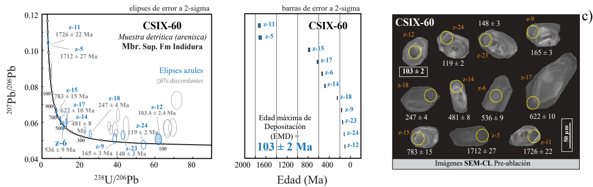
Figura 11 Edades U-Pb en la arenisca clave CSIX-60. a) Gráfico de concordia tipo Tera Wasserburg mostrando todos los datos de los granos de circón analizados, las elipses de color gris representan granos de circón más discordantes, plomo común y/o pérdida de plomo; b) gráfico con las edades más próximas a la edad ^{206}\text{Pb}/^{238}\text{U} máxima de deposición de 103 \pm 2 Ma.; c) imágenes de catodoluminiscencia de granos de circón de la muestra obtenidos por SEM, también se observa el punto de ablación donde se llevó a cabo cada análisis.
