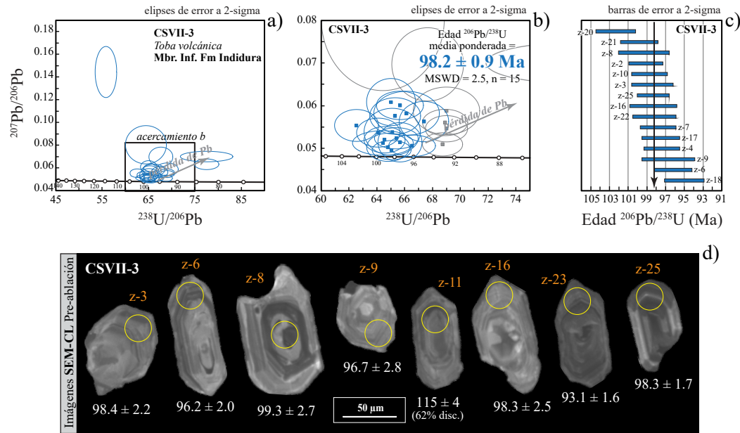
Figura 5. Edades U-Pb en la muestra clave CSVII-3. a) Gráfico de concordia tipo Tera Wasserburg mostrando todos los datos de los granos de circón analizados; b) Esta imagen corresponde a un acercamiento del gráfico a, en ella se muestra la edad ^{206}\text{Pb}/^{238}\text{U} media ponderada de 98.2 \pm 0.9 Ma; c) Gráfico con el número de granos de circón utilizados para calcular la media ponderada; d) Imágenes de catodoluminiscencia de granos de circón representativos con formas subhedrales y núcleos heredados.
