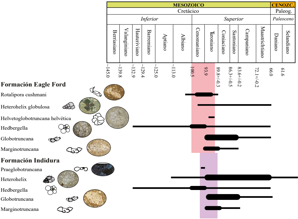
Figura 2. Edad bioestratigráfica calculada a partir del registro de foraminíferos planctónicos presentes en las Formaciones Eagle Ford e Indidura. El miembro superior está marcado por la aparición de la Helvetoglobotruncana helvética y en el miembro inferior por la presencia de la Praeglobotruncana del Cenomaniano tardío.
