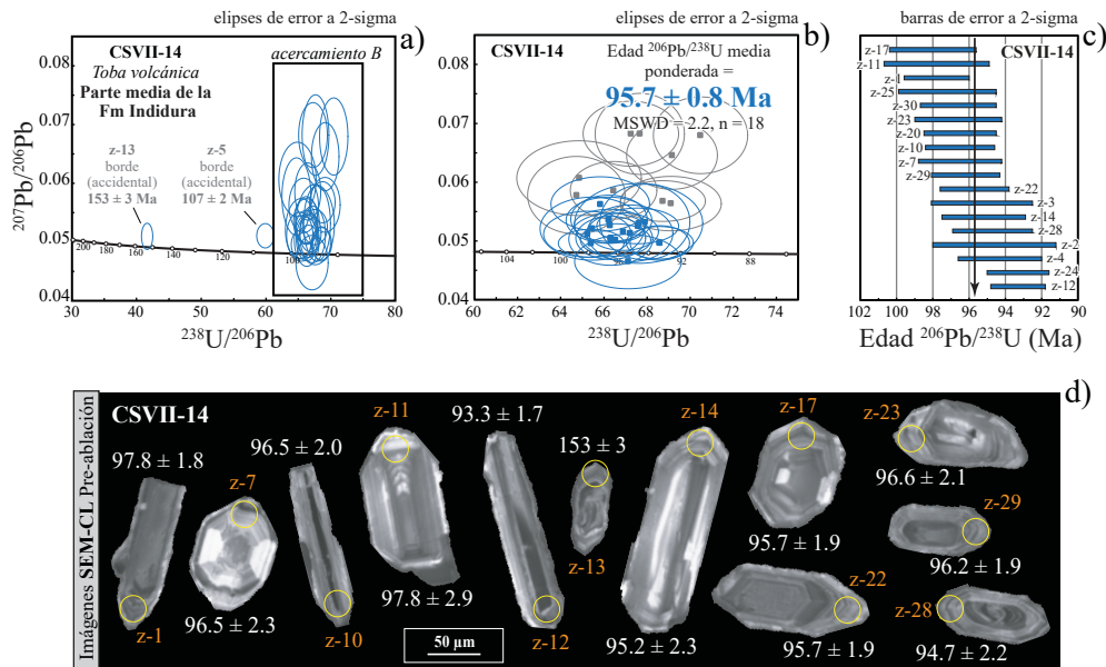
Figura 6 Edades U-Pb en la muestra clave CSVII-14. a) Gráfico de concordia tipo Tera Wasserburg mostrando todos los datos de los granos de circón analizados; b) Esta imagen corresponde a un acercamiento del gráfico a, en ella también se muestra la edad ^{206}\text{Pb}/^{238}\text{U} media ponderada de 95.7 \pm 0.8 Ma. Las elipses de color azul son las que fueron empleadas para calcular la edad media ponderada. c) Gráfico de las edades de los 15 granos de circón utilizados para calcular la media ponderada de 95.7 \pm 0.8 Ma; d) Imágenes de catodoluminiscencia de granos de circón con formas subhedrales alargados y sus anillos de crecimiento.
