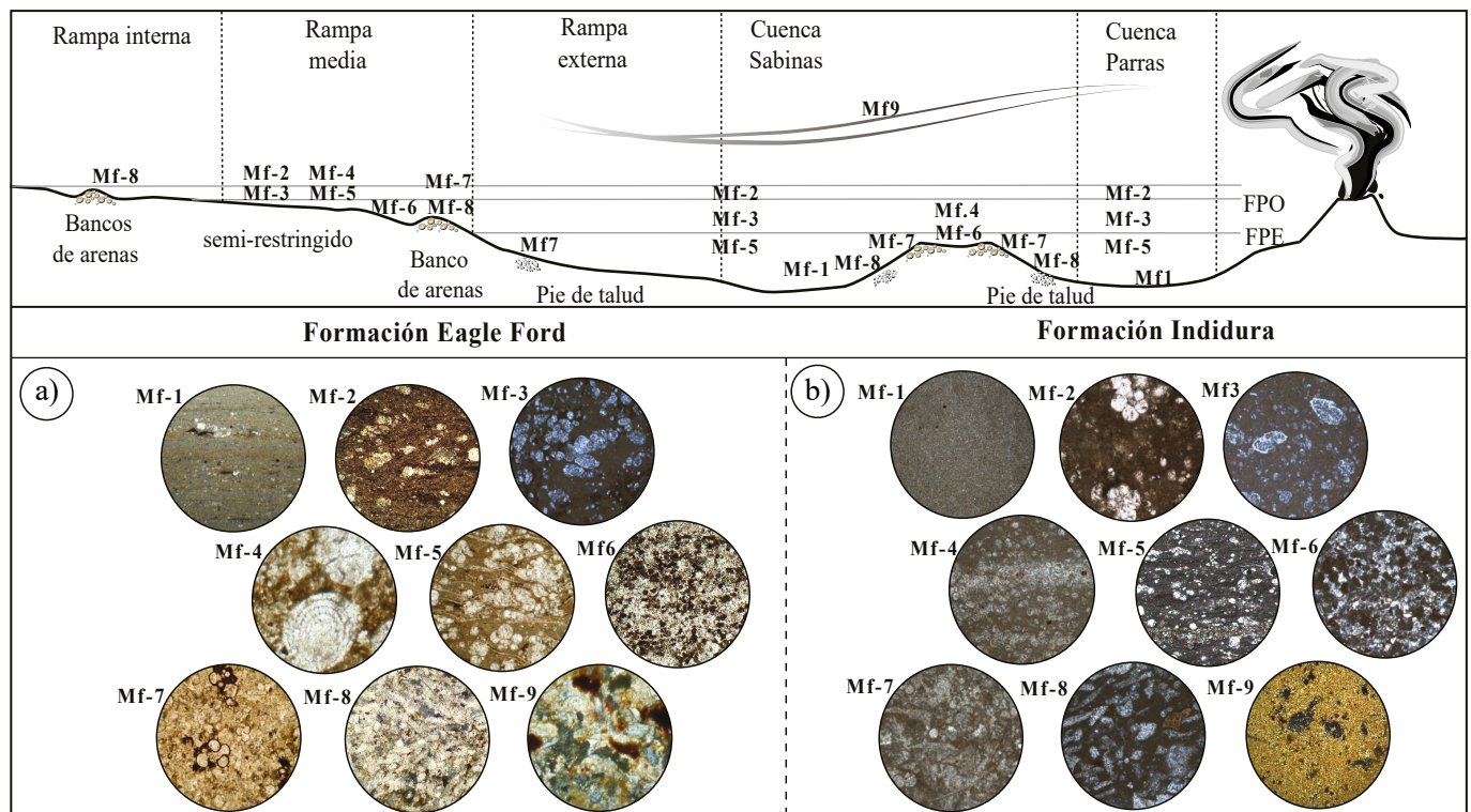
Figura 3. Esta imagen muestra la posición de cada una de las microfacies en el ambiente de depósito de las Formaciones Eagle Ford e Indidura durante el Cenomaniano-Turoniano. Las fotografías se observan en nicols paralelos y muestran los organismos característicos de cada microfacies. Mf-1 mudstone con <10% de aloquímicos, Mf-2 con FP oportunistas, Mf-3 con FP especialistas, Mf-4 con radiolarios y calciesferas, Mf-5 con filamentos, Mf-6 con peloides, Mf-7 con bioclastos, Mf-8 con líticos calcáreos y Mf-9 con cristales de cuarzo y líticos volcánicos.
