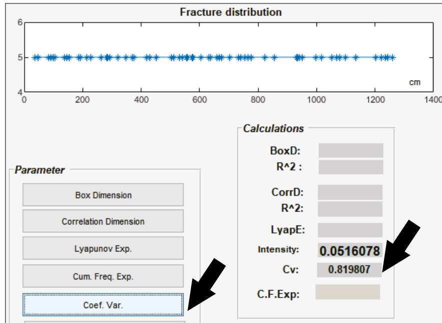
Figura 8. Estimación del coeficiente de variación de un grupo de fracturas (espaciamentos) dando click en el botón Coef. Var.
