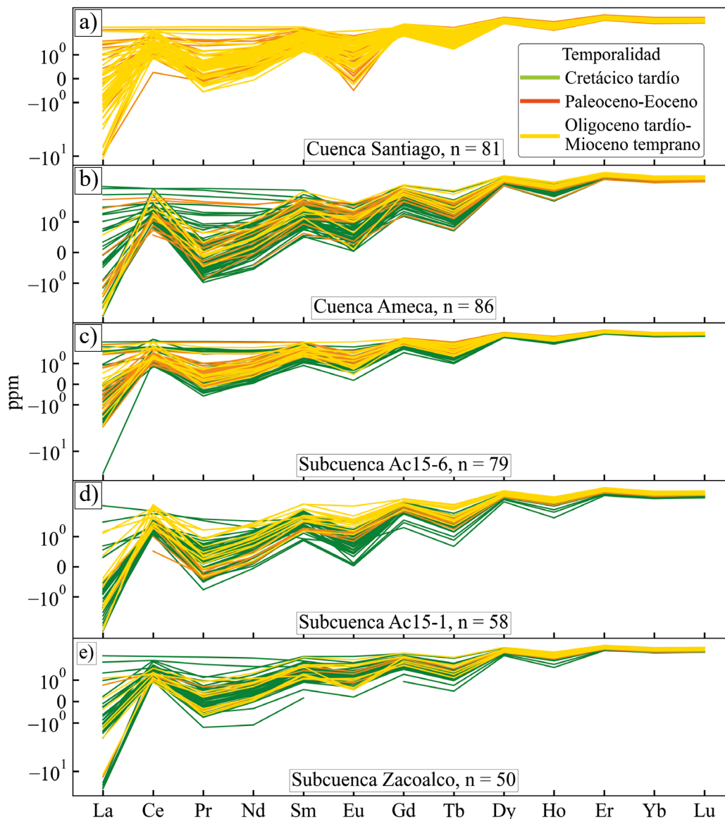
Figura 6. Concentraciones de los ETR normalizadas con las concentraciones de ETR en las condritas (Taylor y McLennan, 1981).
