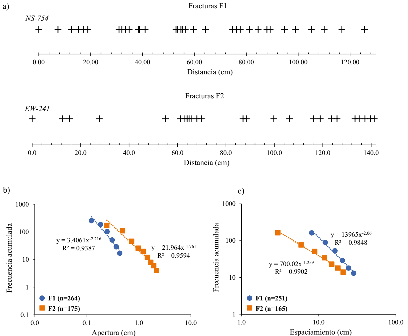
Figura 6. a) Ejemplos de arreglos de fracturas observados en las dos familias de fracturas estudiadas (F1 y F2). b) Gráfico bilogarítmico del tamaño de la apertura contra su frecuencia acumulada para las fracturas F1 y F2. c) Gráfico bilogarítmico del espaciamiento entre fracturas contra su frecuencia acumulada para las fracturas F1 y F2. En los gráficos bilogarítmico se incluye el número de datos (n) que se usó para nuestro análisis.
