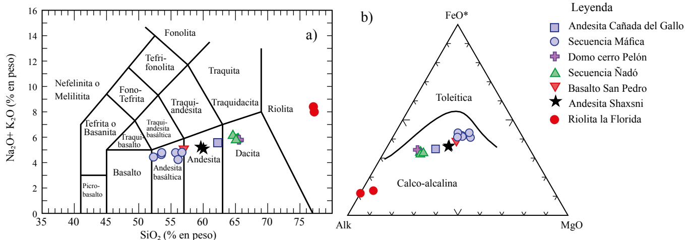
Figura 7. a) Diagrama de álcalis total vs. sílice (Le Bas et al. , 1986) para la clasificación química de las unidades litológicas del CVN. b) Diagrama AFM en que se observa la clasificación dentro de la serie calco-alcalina para las muestras del CVN. Los datos fueron normalizados normalizados al 100% en base anhidra.
