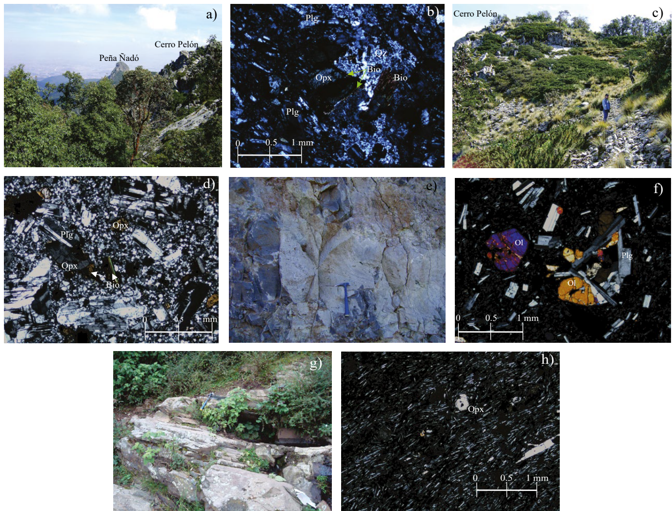
Figura 4. Unidades de la secuencia Ñadó y post-Ñadó. a) Vista panorámica hacia el norte desde la cima del volcán Ñadó, en donde se aprecian la Peña Ñadó y el domo Cerro Pelón. b) Microfotografía de la unidad dacita Ñadó (ÑDO-906), en la que se observan intercrecimientos de cuarzo (Qz) y plagioclasa (Plg) y biotita (Bio), fenocristales de plagioclasa (Plg) y ortopiroxeno (Opx) en una matriz de microlitos de plagioclasa y vidrio. c) Fotografía del Cerro Pelón; lava de color gris claro y de estructura masiva. d) Fenocristales euhédricos de plagioclasa (Plg) y ortopiroxeno (Opx) inmersos en matriz microgranular, en la dacita domo Cerro Pelón (ÑDO-0914). Nótese la presencia de biotita en los bordes del ortopiroxeno. e) Fotografía de un afloramiento correspondiente al vulcanismo máfico, en donde se observa un derrame de lava masiva, emitido por un cono de escoria. f) Microfotografía que muestra la textura porfídica, con fenocristales de olivino (Ol) y plagioclasa (Plg) embebidos en una mesostasis de microlitos de plagioclasa y vidrio de productos del vulcanismo máfico (ÑDO-0926). g) Fotografía de un afloramiento de la unidad Cañada del Gallo, el cual presenta lavas con una estructura lajeada, de color gris claro. h) Microfotografía de la andesita Cañada del Gallo. Se observan fenocristales subédricos de ortopiroxeno (Opx) inmersos en una mesostasis constituida por microlitos de plagioclasa orientados (ÑDO-0911).
