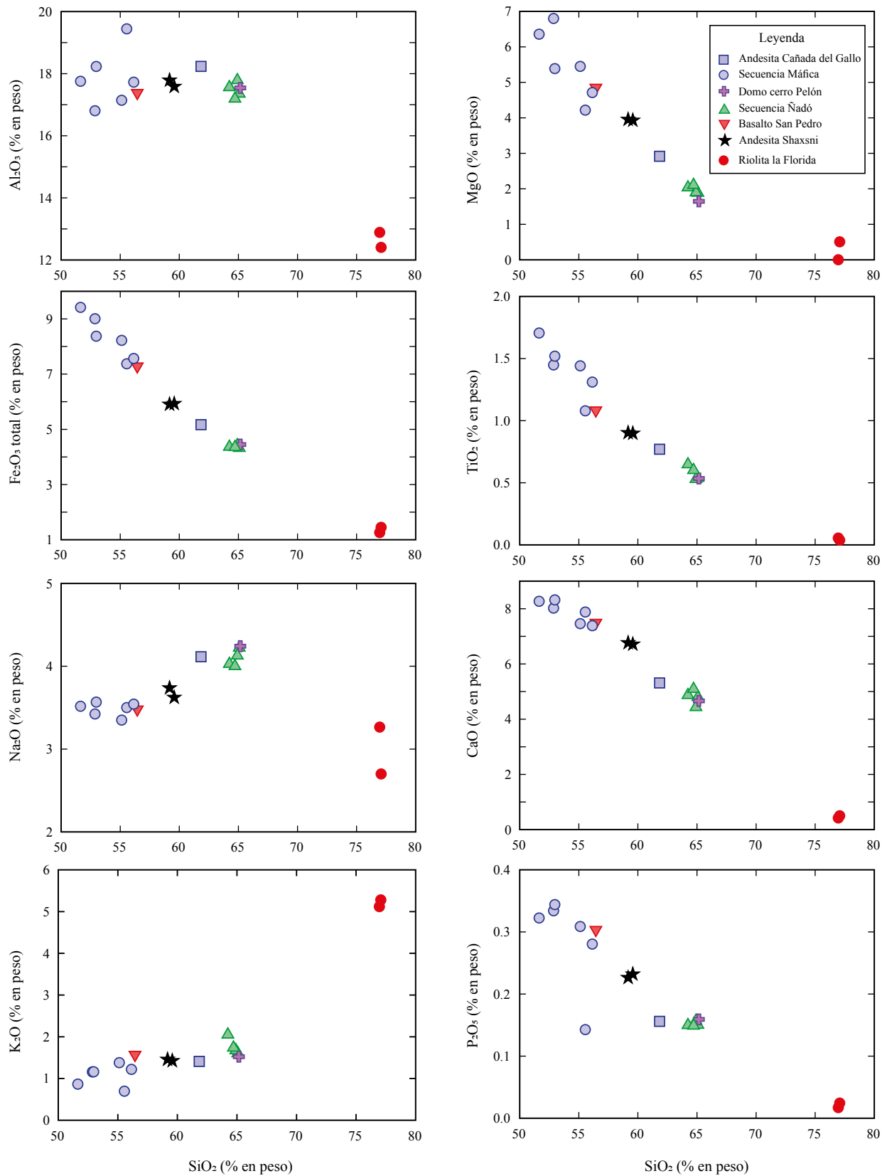
Figura 8. Diagramas de Harker de los elementos mayores vs. SiO 2 (% en peso) para las rocas del CVN. Los datos fueron normalizados al 100% en base anhidra y el Fe total se reporta como Fe 2 O 3 .
