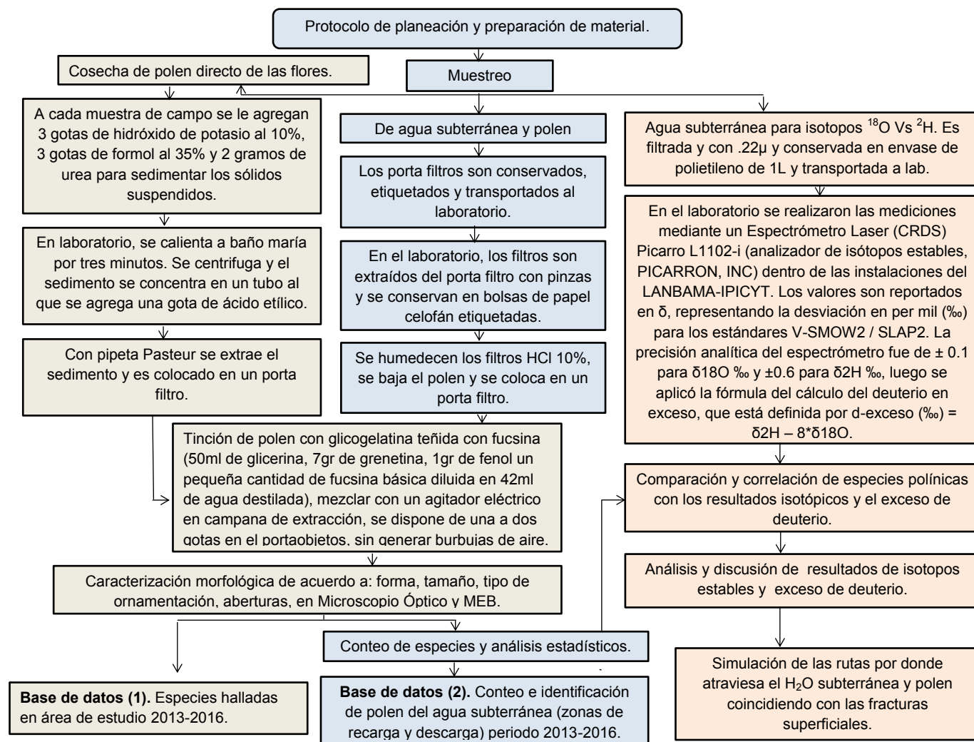
Figura 3. Diagrama de flujo de la metodología polínica ambiental (MEPAM).
