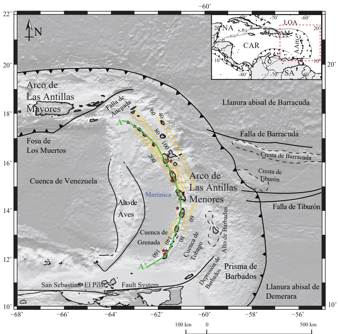
Figura 1. Rasgos tectónicos cercanos al arco de las Antillas Menores. En la esquina superior derecha se presenta el área de estudio dentro del contexto de la placa del Caribe. Las abreviaciones simbolizan: NA, Placa Norteamericana; SA, Placa Suramericana; CAR, Placa del Caribe; LOA, Litósfera Oceánica del Atlántico; AAM, Arco de las Antillas Mayores; AAm, Arco de las Antillas Menores. Las estrellas rojas representan los volcanes con actividad relativamente reciente (Bouysse et al. , 1990). Las líneas amarillas punteadas representan la profundidad de la losa de subducción cada 20 km (Bouysse y Westercamp, 1988). La línea verde (A-A') representa la ubicación del modelo presentado en la Figura 8.
