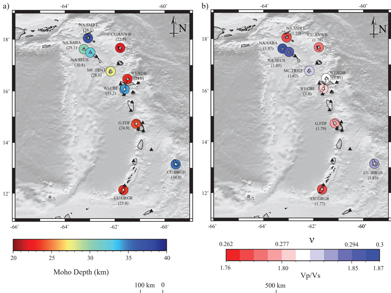
Figura 7. Representación espacial de los resultados obtenidos con el análisis de funciones receptoras: (a) profundidad de Moho estimada para las distintas estaciones; (b) relación V_p/V_s o coeficiente de Poisson ( \nu ) para las distintas estaciones.
