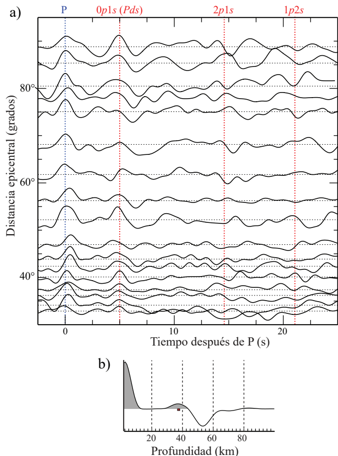
Figura 3. Ejemplo de funciones receptoras para la estación NA.SABA generadas a partir de las componentes radial y vertical de los sismogramas. (a) Funciones receptoras en tiempo ordenadas por la distancia epicentral en grados. La línea vertical azul marca la llegada de la onda P, las líneas rojas marcan la llegada aproximada de las distintas fases convertidas para una corteza de 29 km de espesor. La más evidente y coherente de éstas es la llegada de la fase Pds (b) Función receptora después de apilada en profundidad. El cuadro rojo representa la profundidad seleccionada para la profundidad de Moho.
