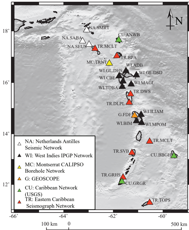
Figura 2. Estaciones sismológicas en las Antillas Menores. Los distintos colores representan las diferentes redes sismológicas que se encuentran actualmente activas en esta región. De las 25 estaciones representadas en el mapa, solo nueve pudieron ser utilizadas para aplicar la técnica de funciones receptoras.
