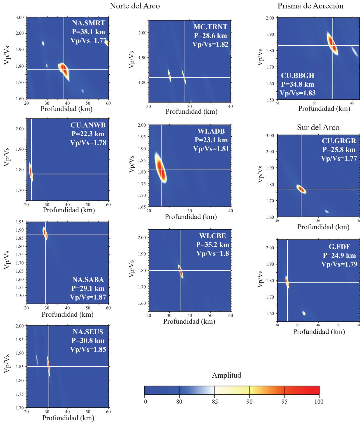
Figura 6. Todos los análisis H- \kappa para las estaciones. La cruz blanca marca la proyección del máximo valor de amplitud a los ejes de profundidad y relación Vp/Vs .
