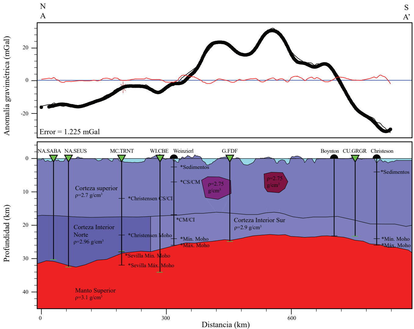
Figura 8. Modelo gravimétrico directo a lo largo del eje del arco de las Antillas Menores. Solo la componente regional es modelizada para verificar las estimaciones de la profundidad de la discontinuidad de Moho en el arco. En la anomalía, la línea negra gruesa representa la anomalía regional observada; la línea delgada representa la respuesta del modelo; y la línea roja, el error del modelo (Error total = 1.225 mGal). Los polígonos azules representan las zonas de agua. Las líneas verticales representan algunas de las estimaciones de profundidad existentes en el arco proyectadas al perfil. Los triángulos verdes representan la localización de las estaciones sísmológicas utilizadas en este estudio, mientras que los semicírculos negros representan la posición de las líneas sísmicas perpendiculares a éste. Los nombres en el modelo simbolizan la fuente de la profundidad representada: Boynton (Boynton et al. , 1979), Christensen (Christensen, 2009), Christeson (Christeson et al. , 2008), Sevilla (Sevilla et al. , 2010) y Weinzierl (Weinzierl, 2010). Las abreviaturas simbolizan: CS/CM, discontinuidad corteza superior-corteza intermedia; CM/CI, discontinuidad corteza intermedia-corteza inferior; Mín. Moho, mínimo valor del Moho; Máx. Moho, máximo valor del Moho.
