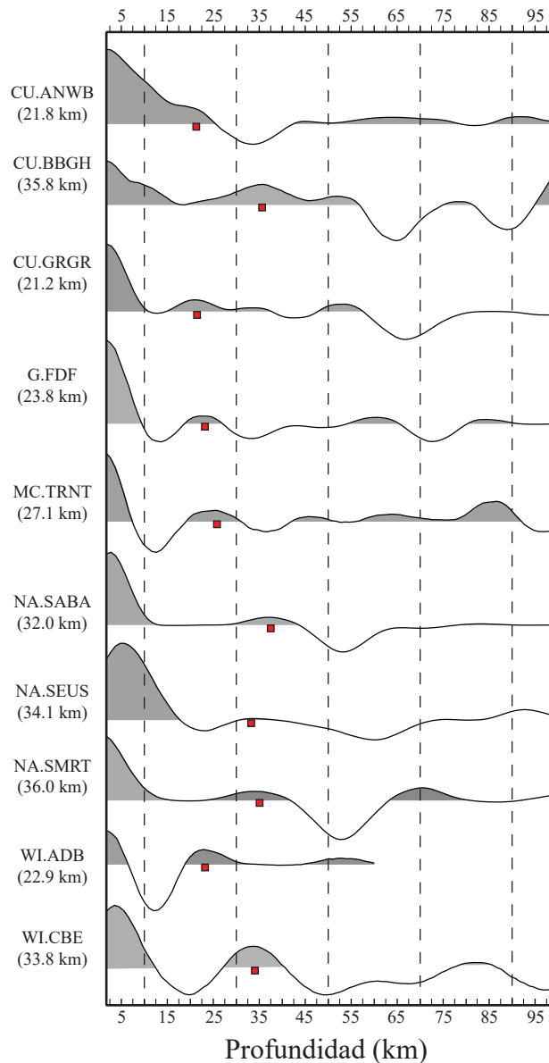
Figura 4. Funciones receptoras apiladas en profundidad para todas las estaciones. El cuadro rojo representa la profundidad seleccionada para la interfaz de Moho.
