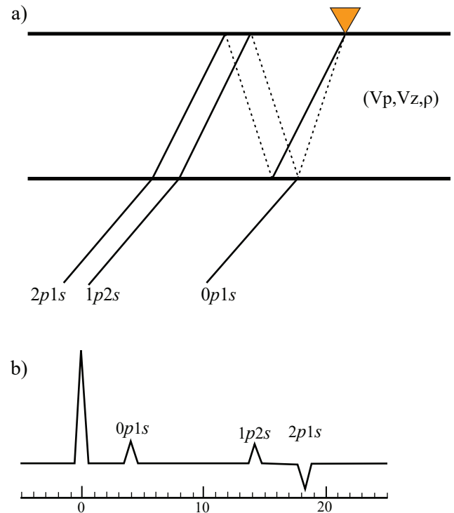
Figura 5. (a) Caminos de la onda P directa, la onda PdS y las reverberaciones para un modelo de una capa. En la notación utilizada (NpMs), N y M corresponden al número de segmentos p y s en el camino del rayo dentro de la corteza. (b) Función receptora (de la componente radial) teórica mostrando las llevadas de las distintas reverberaciones para un modelo de una capa basado en el iasp91.
