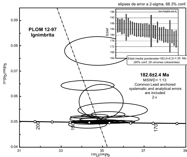
Figura 11. Diagrama de concordia tipo Tera-Wasserburg para los resultados de la muestra PLOM-12-97. En el recuadro el diagrama de barras de error se muestra la edad media de 183.3 \pm 0.31 - 1.35 Ma.
