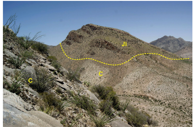
Figura 14. Limolitas, brechas y areniscas rojas del Jurásico Inferior (Ji) descansan de forma discordante sobre calizas paleozoicas del Carbonífero (C) en el cañón Sartorios, al noroeste de la mina La Chona.
