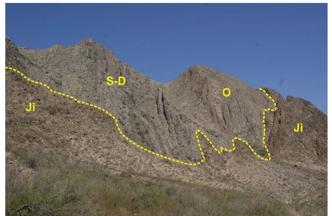
Figura 16. Brechas y conglomerados del Jurásico Inferior (Ji) fuertemente basculados descansan de forma discordante sobre calizas polideformadas del Paleozoico Inferior (Ordovícico (O), Silúrico (S) y Devónico (D)) en el flanco noreste del Cerro de Enmedio. La línea punteada señala la discordancia angular y erosional de las capas jurásicas sobre la sucesión del Paleozoico Inferior.
