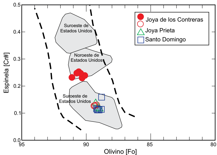
Figura 6. Gráfico que muestra la relación entre Mg# y Cr# en algunos xenolitos del grupo Santo Domingo. En la gráfica se aprecia que éstos caen adentro del arreglo del manto (líneas punteadas) propuesto por Arai (1994). Las zonas en gris representan peridotitas del oeste de los Estados Unidos (Kil y Wendlandt, 2004, Titus, et al. , 2007 y Luffi, et al. , 2009). Los símbolos huecos corresponden a xenolitos sin metasomatismo aparente o modal, los símbolos rellenos son xenolitos con metasomatismo modal. Los símbolos empleados se utilizan en las figuras subsiguientes. Fo\% = (Mg \times 100) / (Mg + Fe) . Cr\# = (Cr \times 100) / (Cr + Al) .
