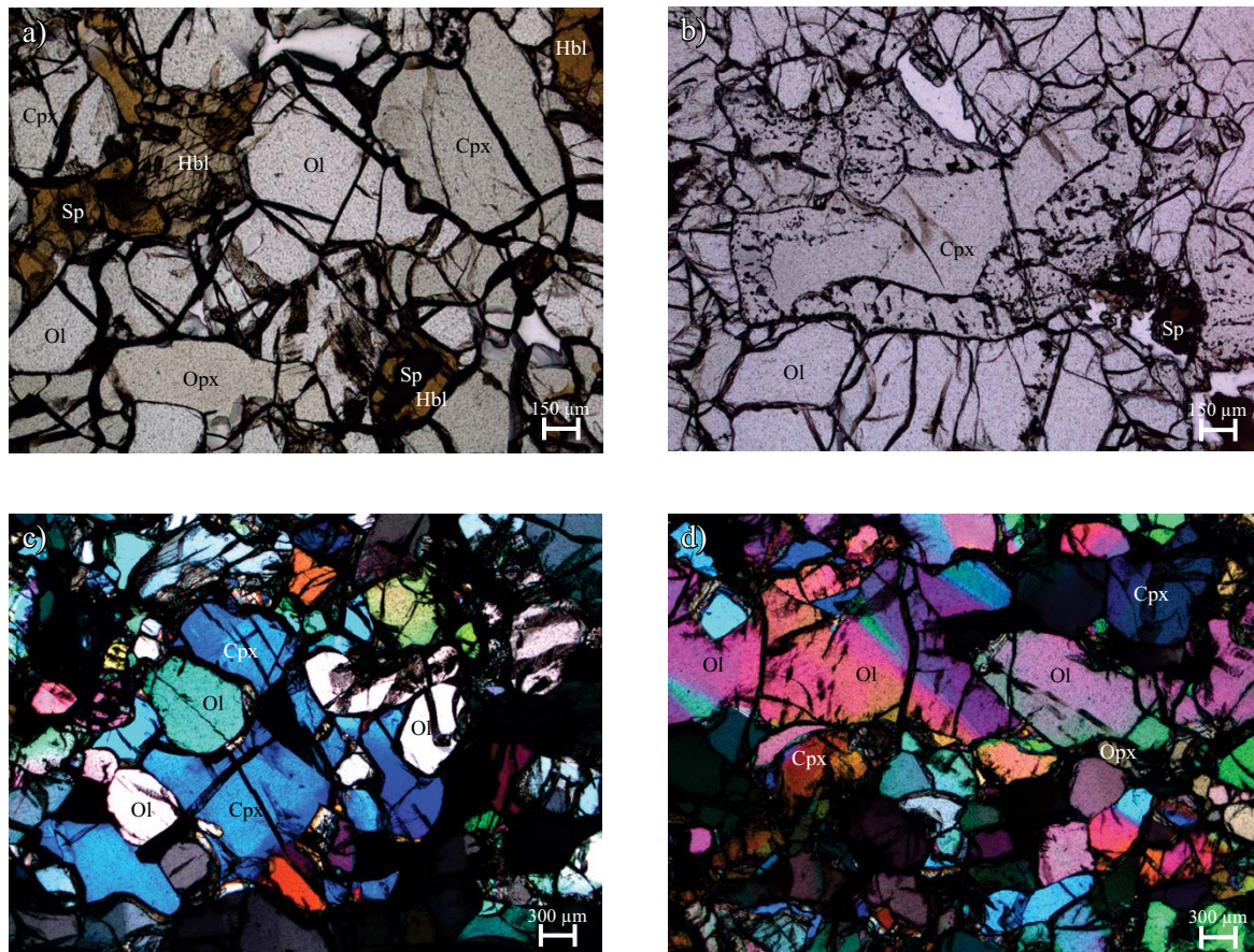
Figura 4. a) Detalle de anfíboles rodeando espinelas, luz plana polarizada (muestra SD7). b) Cristal de clinopiroxeno con textura “esponjosa” y alineamiento de inclusiones fluidas; luz plana polarizada (muestra SD8). c) Porfiroclasto de clinopiroxeno poikilitico; nícoles cruzados (muestra SD11). d) Porfiroclasto de olivino con extinción deformada, nícoles cruzados (muestra SD10). Simbología: Ol, olivino, Opx, ortopiroxeno, Cpx, clinopiroxeno, Sp, espinela, Hbl, hornblenda.
