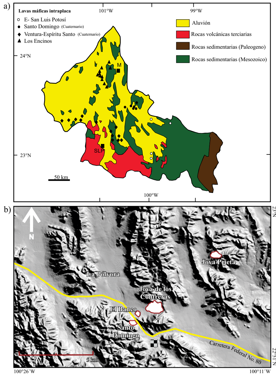
Figura 1. a) Mapa de San Luis Potosí con la geología general y la ubicación de los campos volcánicos de intraplaca. M: Matehuala; SLP: San Luis Potosí. b) Modelo digital de elevación del Campo Volcánico Santo Domingo, señalando los tres maares principales en donde se colectaron los xenolitos investigados: Joya Prieta, Joya de los Contreras y Santo Domingo.
