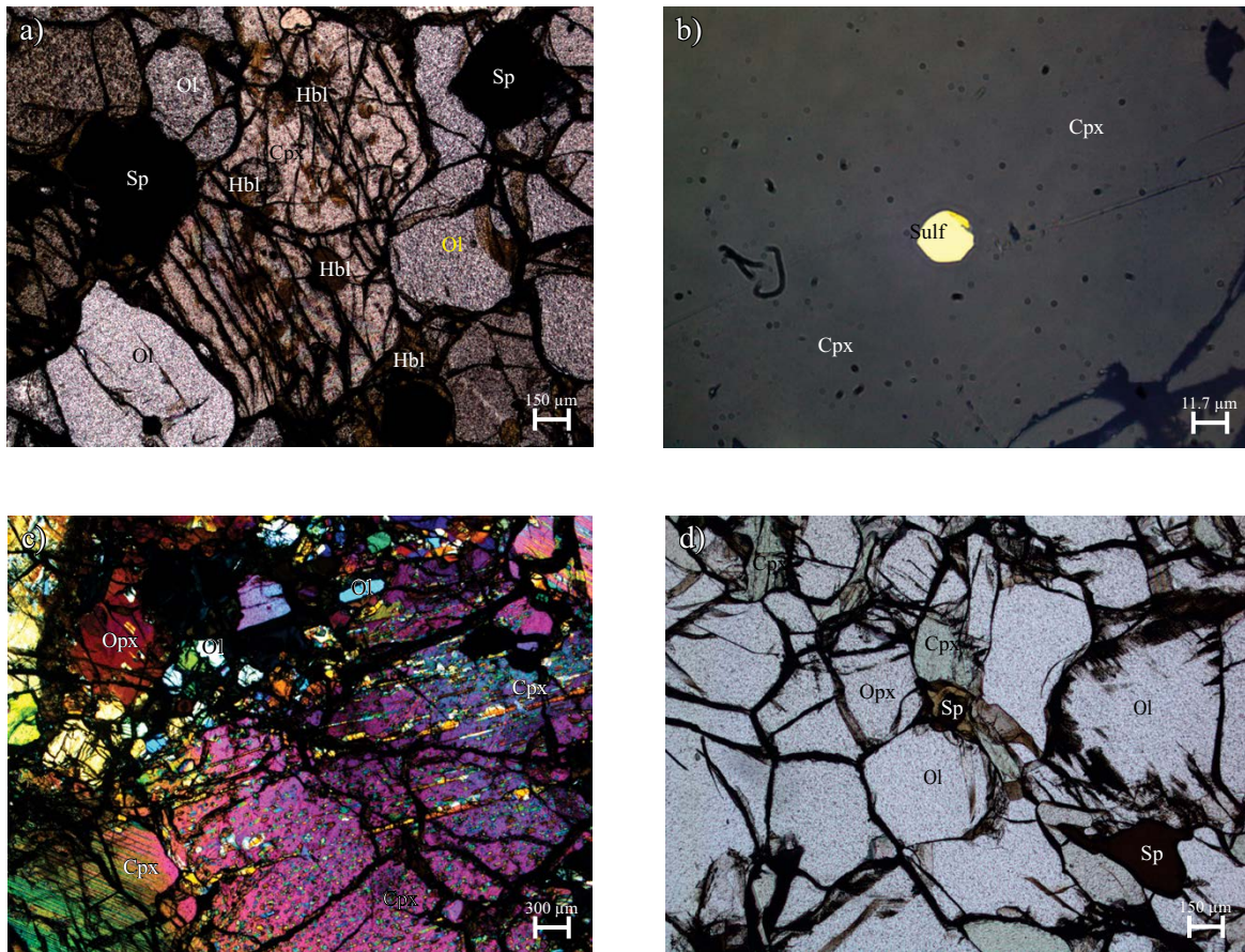
Figura 5. a) Detalle de clinopiroxeno invadido por anfíbol; luz plana polarizada (muestra JP6). b) Gota de sulfuro dentro de clinopiroxeno; luz reflejada (muestra JP2). c) Cristal de clinopiroxeno con lamelas de exsolución en clinopiroxenita (JP1); nicóles cruzados d) Espinela rodeada de anfíbol y a su vez intersticial entre olivinos y piroxenos; luz plana polarizada (muestra JP3). Simbología: Ol, olivino, Opx, ortopiroxeno, Cpx, clinopiroxeno, Sp, espinela, Sulf, sulfuro, Hbl, hornblenda.
