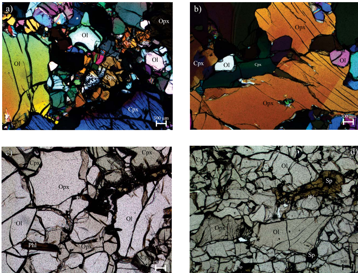
Figura 3. a) Vista general de porfidoclastos de olivino y piroxeno con sus respectivos neoblastos; nicoles cruzados (muestra JC2). b) Porfidoclasto de ortopiroxeno deformado; nicoles cruzados (muestra JC16). c) Detalle de cristales de flogopita, luz plana polarizada (muestra JC13). d) Espinela anédrica rodeada por anfíbol; luz plana polarizada (muestra JC21). Simbología: Ol, olivino, Opx, ortopiroxeno, Cpx, clinopiroxeno, Sp, espinela, Hbl, hornblenda, Phl, flogopita. Nótese que todas las láminas delgadas son de 100 micras de espesor, lo que facilita la identificación de los piroxenos, con base en su color, en luz plana polarizada. Con nicoles cruzados las fases presentan colores anómalos debido al grosor de las láminas.
