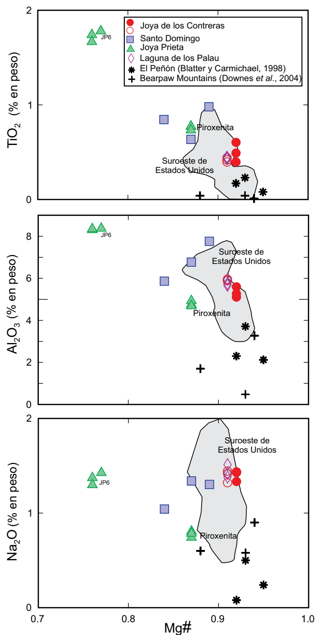
Figura 8. Gráficos de algunos elementos mayores en función del Mg# reportado para los clinopiroxenos analizados del grupo Santo Domingo. Las áreas en gris, representan muestras de clinopiroxeno en peridotitas del suroeste de los Estados Unidos (Kil y Wendlandt, 2004, Titus et al. , 2007 y Luffi et al. , 2009).
