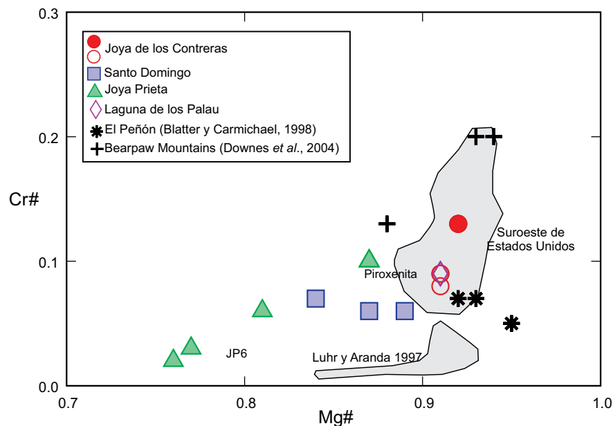
Figura 7. Gráfico de Mg# vs. Cr# en cristales de diópsida para las muestras analizadas del grupo Santo Domingo. Las áreas en gris representan las composiciones de diópsida en peridotitas del suroeste de los Estados Unidos (Kil y Wendlandt, 2004, Titus, et al. , 2007 y Luffi, et al. , 2009) y en algunas muestras mexicanas estudiadas por Luhr y Aranda-Gómez (1997). Así mismo, se incluyen análisis de muestras metasomatizadas de la región de El Peñón (Blatter y Carmichael, 1998), en el Cinturón Volcánico Mexicano. Mg\# = (Mg \times 100) / (Mg + Fe) . Cr\# = (Cr \times 100) / (Cr + Al) .
