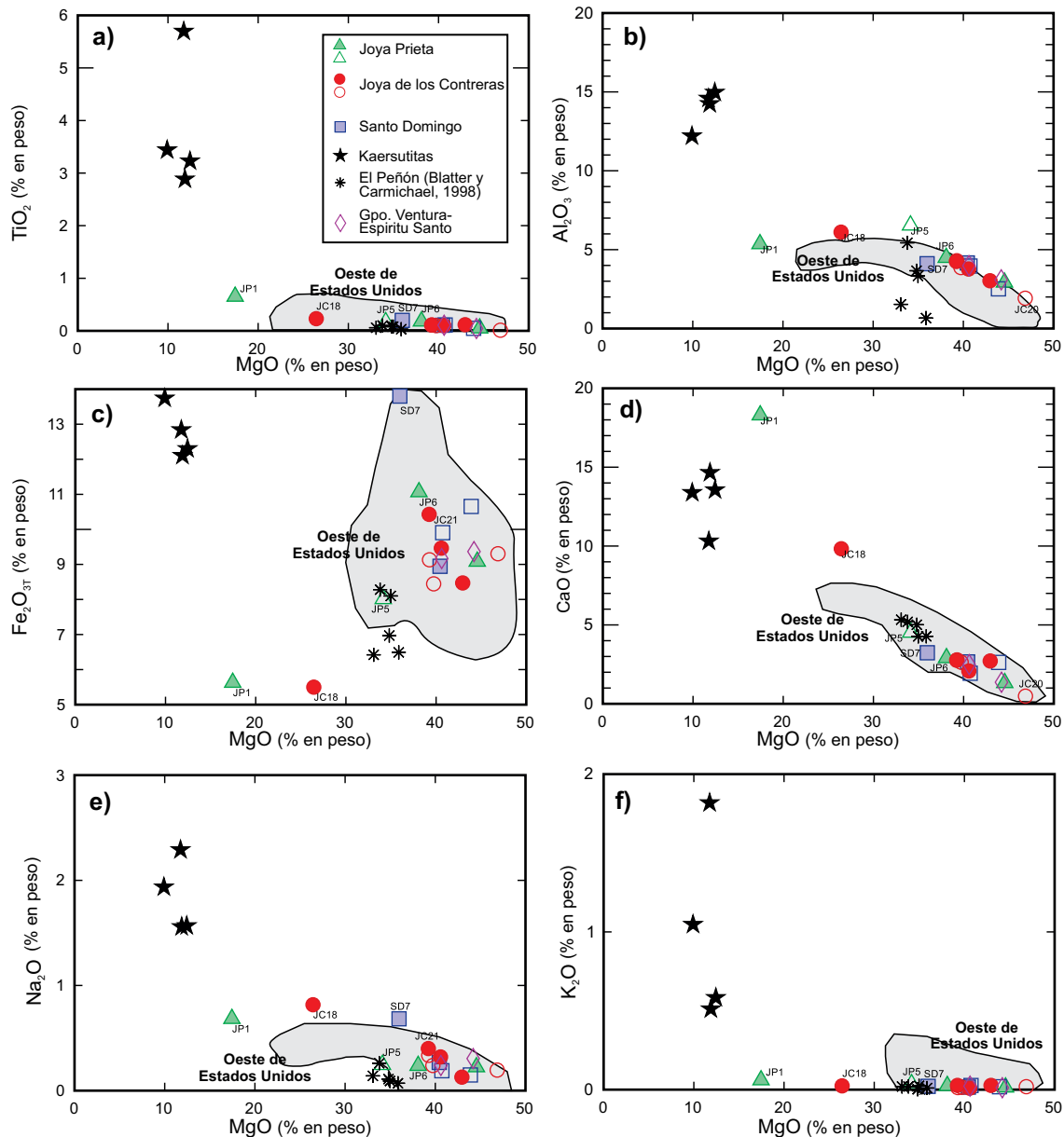
Figura 12. Diagramas de variación de algunos elementos mayores con respecto al contenido de MgO. Los símbolos huecos corresponden a xenolitos sin metasomatismo modal aparente, los símbolos rellenos son xenolitos con metasomatismo modal inferido a partir de la presencia de anfíbol y/o flogopita. Las áreas en gris representan xenolitos del manto del oeste de los Estados Unidos.
