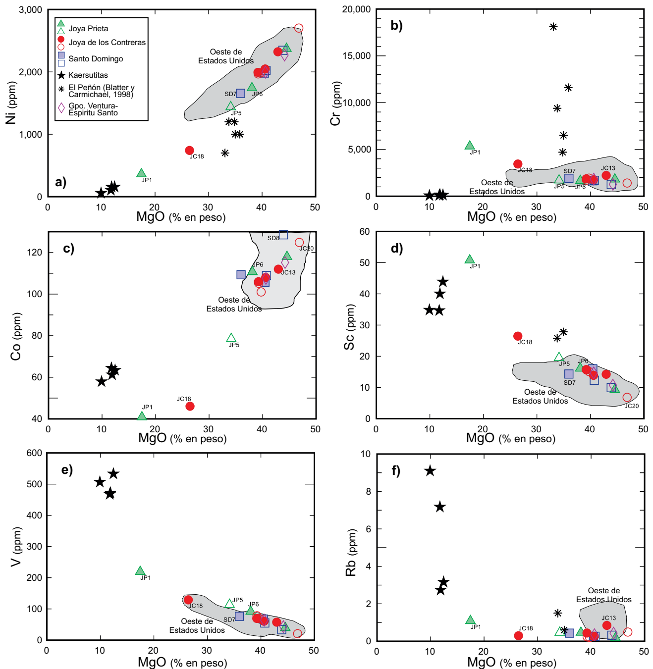
Figura 13. Diagramas de variación de algunos elementos traza, en ppm, con respecto al contenido de MgO, en % en peso. Los símbolos huecos corresponden a xenolitos sin metasomatismo modal aparente, los símbolos rellenos son xenolitos con metasomatismo modal inferido a partir de la presencia de anfíbol y/o flogopita. Las áreas en gris representan xenolitos del manto del oeste de los Estados Unidos.
