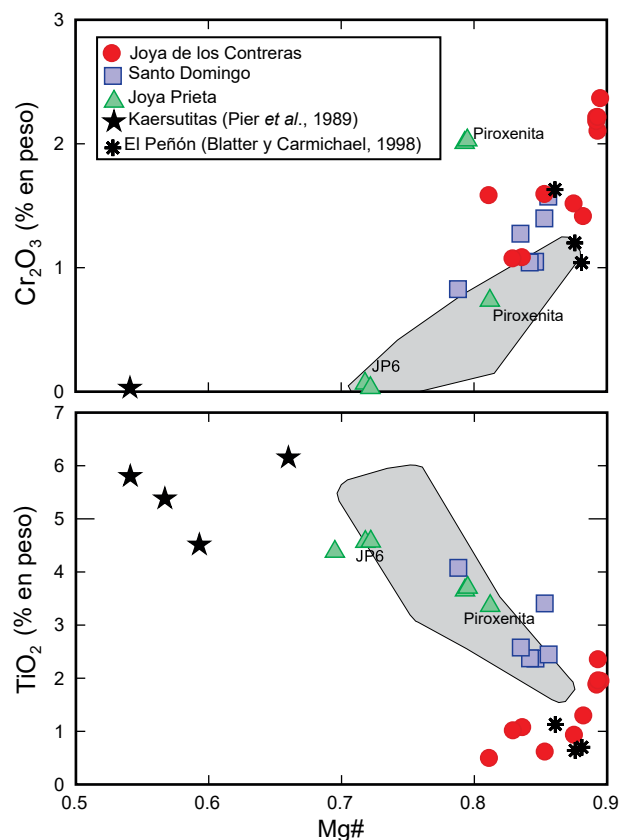
Figura 9. Gráficos del contenido de \text{TiO}_2 y a \text{Cr}_2\text{O}_3 en función del Mg# en anfíbol. Las áreas en gris representan muestras estudiadas en la región oeste de los Estados Unidos.
