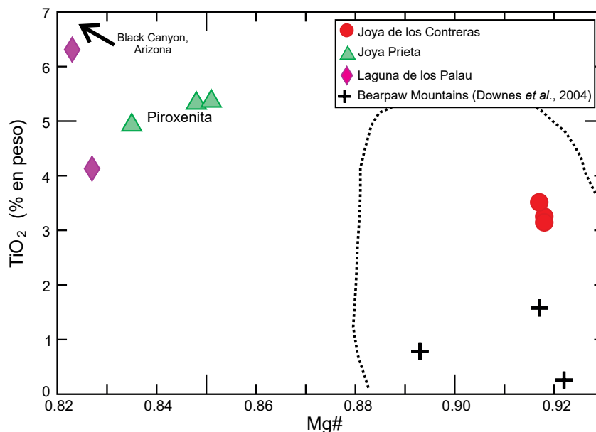
Figura 10. Gráfico de TiO 2 en flogopita en función del Mg# en peridotitas del manto. El área limitada por la línea punteada corresponde al arreglo del manto propuesto por McDonough y Rudnick (1998). Se incluye la composición de flogopitas reportadas por Luhr y Aranda-Gómez (1997) en una lherzolita proveniente de uno de los volcanes del grupo Ventura-Espíritu Santo. Nótese que las flogopitas del grupo Santo Domingo presentan dos composiciones distintas, dependiendo de si se encuentran en lherzolita o en piroxenita.
