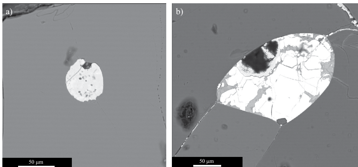
Figura 11. a) Gota de sulfuro tipo mss intracristalino en olivino. b) Bleb tipo mss intercristalino entre clinopiroxeno y olivino. Nótese la presencia de hematita por oxidación.
