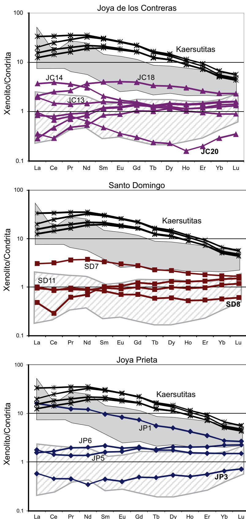
Figura 14. Diagramas de tierras raras normalizadas a condrita (Nakamura, 1974) de todos los xenolitos estudiados, se comparan con lo reportado para El Peñón (Mukasa et al. , 2007), representado en la zona gris. La zona con patrón en diagonal representa muestras de peridotita reportadas en el suroeste de los Estados Unidos.
