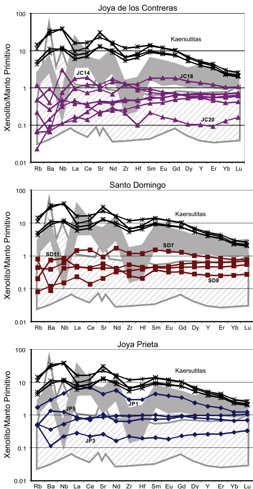
Figura 15. Diagramas de elementos traza normalizados con los valores del manto primitivo (Sun y McDonough, 1989) que engloba todos los xenolitos estudiados; se comparan con lo reportado en El Peñón (Mukasa et al. , 2007), representado en la zona gris. La zona con patrón en diagonal representa muestras de peridotita reportadas en el suroeste de los Estados Unidos.
