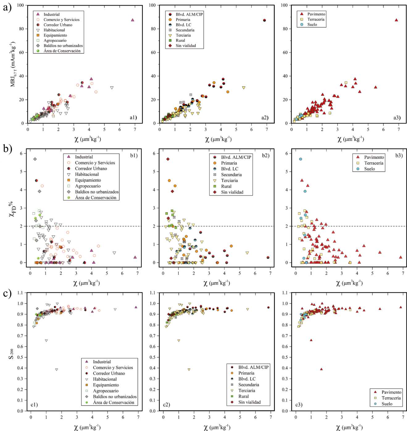
Figura 4. Diagramas de dispersión para a) MRI 0.7T versus \chi , b) \chi_{FD}\% versus \chi , y c) S_{200} versus \chi con discriminación de puntos según: a1-b1-c1) uso de suelo; a2-b2-c2) tipo de vialidad; a3-b3-c3) superficie de barrido del polvo.
