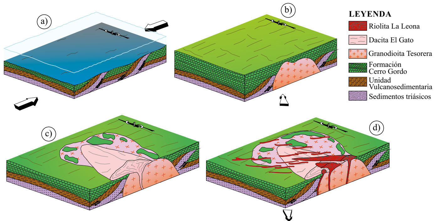
Figura 13. Modelos esquemáticos propuestos para el emplazamiento de los diques y domos riolíticos, influenciado por la evolución tectónica regional. a) Acreción del terreno Guerrero con el terreno Sierra Madre, formando fallas de cabalgaduras. b) Intrusión de la Granodiorita Tesorera en las capas de caliza previamente deformadas. c) Emplazamiento de la dacita El Gato formando estructuras dómicas amplias. d) Emplazamiento de diques y domos riolíticos La Leona, durante las primeras etapas de extensión NE-SW cortan a los cuerpos intrusivos, a la dacita y a los sedimentos marinos con orientación NW-SE.
