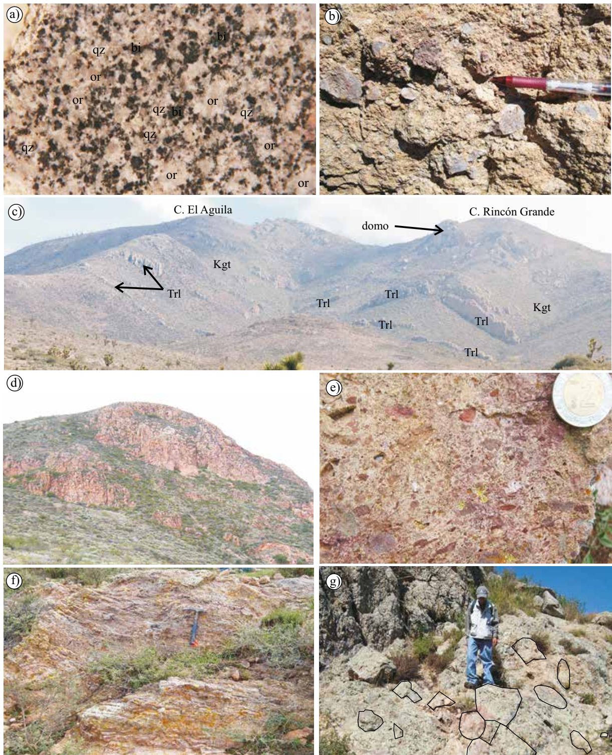
Figura 4. Compendio de imágenes que muestran algunos detalles de las diferentes unidades que forman la estratigrafía local del área del CIT. a) Textura porfirítica de la Granodiorita Tesorera, observándose fenocristales de cuarzo (qz), ortoclasa (or) y biotita (bi), muestra colectada en la localidad de Noria del Cerro, coordenadas UTM 796,150-2'519,893. b) Brecha basal de desintegración de la dacita El Gato, donde se aprecia la dacita autobrechada, con fragmentos ~4 cm (fotografía tomada en el C. Salto El Gato). c) Panorámica que muestra el sistema de diques de la riolita La Leona, emplazados en la Granodiorita Tesorera en los cerros El Águila y Rincón Grande, sistema de diques en un arreglo paralelo de orientación NW-SE, remanente de un domo en el cerro Rincón Grande, Granodiorita Tesorera (Kgt), riolita La Leona (Trl; Panorámica viendo al norte). d) domo Cerro Colorado, emplazado sobre la margen oriental de la granodiorita Tesorera. e) Derrame piroclástico basal de la riolita La Cardona, contenido alto de líticos alargados y angulosos de 2 cm de largo; afloramiento al sur del cerro Piedras de Amolar en la zona de contacto con un techo colgante de la Formación Cerro Gordo. f) Afloramiento en el lecho del arroyo al sur del cerro Piedras de Amolar, observándose estructura fluidal con ligera oxidación que corresponde a la riolita La Cardona. g) Brecha de rezag, con fragmentos de hasta 50 cm de diámetro de la ignimbrita San Patricio, asociado a una fuente de emisión cercana; afloramiento localizado aguas arriba del Arroyo San Patricio.
