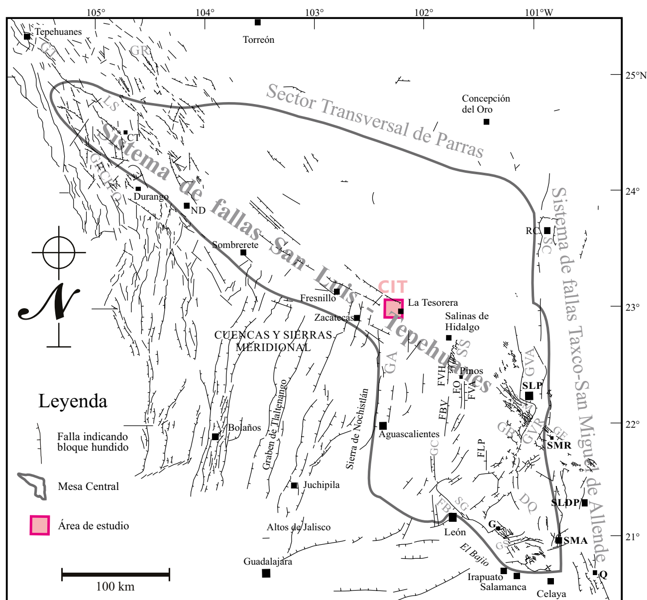
Figura 5. Ubicación del CIT, dentro del Sistema de Fallas San Luis-Tepehuanes en el tramo Salinas de Hidalgo-Zacatecas, al suroriente se localiza la zona de Cuencas y Sierras meridional (modificado de Nieto-Samaniego et al. , 2005).
