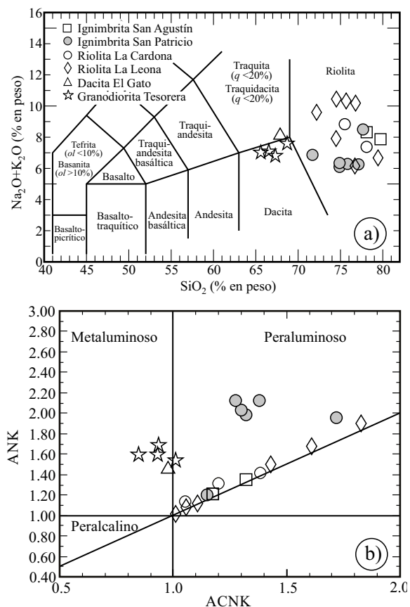
Figura 9. Diagramas geoquímicos de elementos mayores de las unidades volcánicas del Complejo Volcánica La Tesorera. a) Diagrama de elementos alcalinos totales vs. sílice (LeBas et al. , 1986); q: cuarzo; ol: olivino normativos. b) Diagrama de saturación de alúmina de las unidades volcánicas del CIT.
