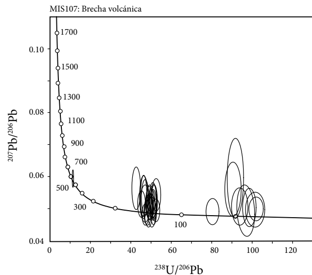
Figura 13. Diagrama de concordia Tera-Wasserburg mostrando las poblaciones de edad de la brecha volcánica de Mezquitlán (MIS107) perteneciente a la Formación Tetelcingo (18°2'3.11"N, 98°56'17.66"W).
