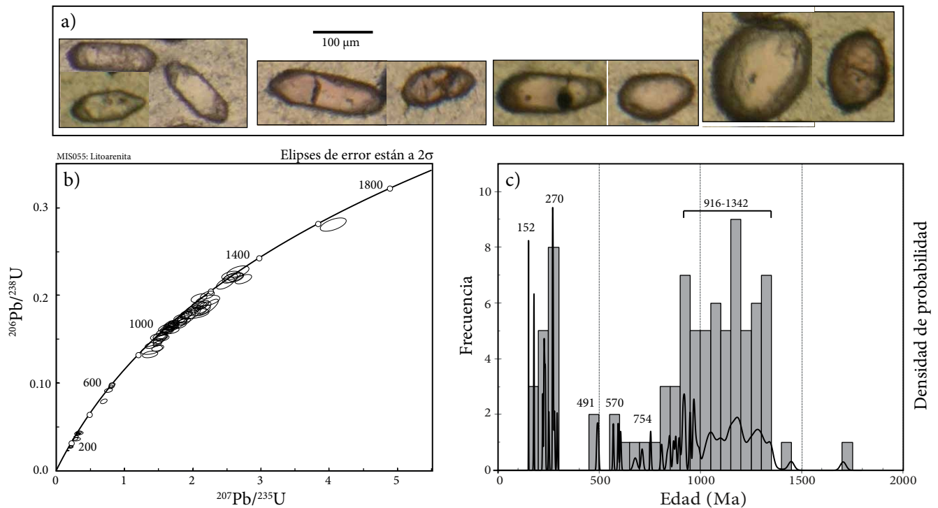
Figura 11. Geocronología de circones detríticos de litoarenita de la localidad San Juan de las Joyas, Miembro Ajuatetla ( 17^{\circ}45'35.50''\text{N} , 99^{\circ}5'10.65''\text{W} ). a) Características de las cuatro familias morfológicas de circones; b) Diagrama de concordia Wetherill mostrando las edades de los circones detríticos de la muestra MIS055; c) Diagrama de densidad de probabilidad para las edades de los circones detríticos de la muestra MIS055. Todos los errores tienen una desviación estándar de 2\sigma .
