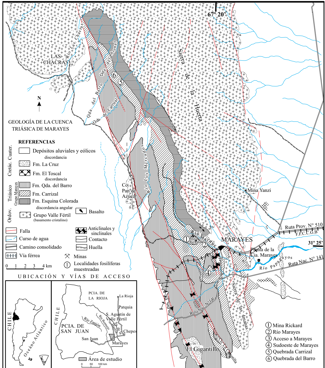
Figura 1. Mapa de ubicación de la Cuenca de Marayes-El Carrizal. Modificado de Bossi (1976).
