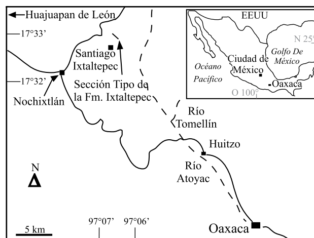
Figura 1. Localización geográfica de la Formación Ixtaltepec en su sección tipo, Arroyo Las Pulgas, donde fueron colectados los ejemplares de braquiópodos productidos.
