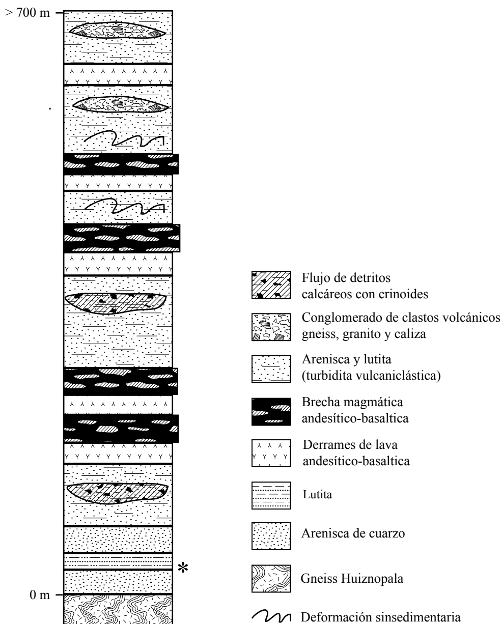
Figura 2. Columna estratigráfica de la Formación Tuzancoa. El asterisco indica el nivel de procedencia del material descrito (Modificado de Rosales-Lagarde, 2002).
