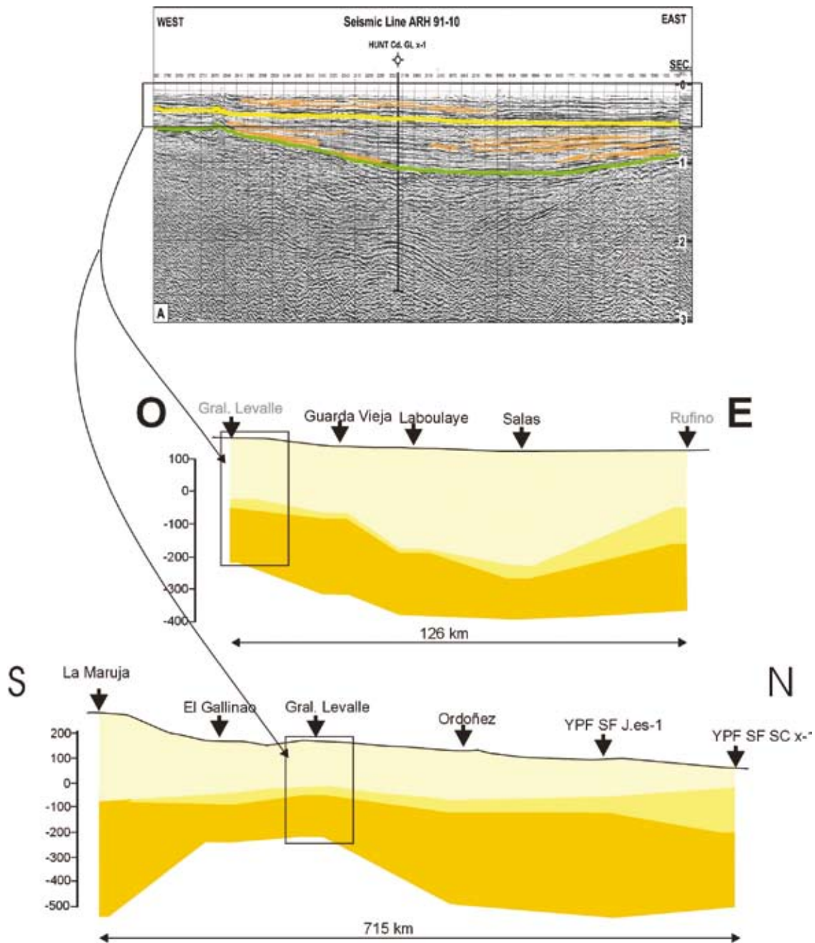
Figura 11. Secciones geológicas regionales, norte-sur y este-oeste del Cenozoico del subsuelo de la Llanura Pampeana (modificada de Marengo 2006). Los distintos tonos señalan los paquetes del Mioceno inferior (más oscuro), medio y superior (más claro). El paquete intermedio (Mioceno medio) representa los estratos marinos de la Fm Paraná. Los rectángulos muestran la ubicación de la sección sísmica ARH 91 (modificada de Webster et al. 2004) en el marco regional de la Llanura.
