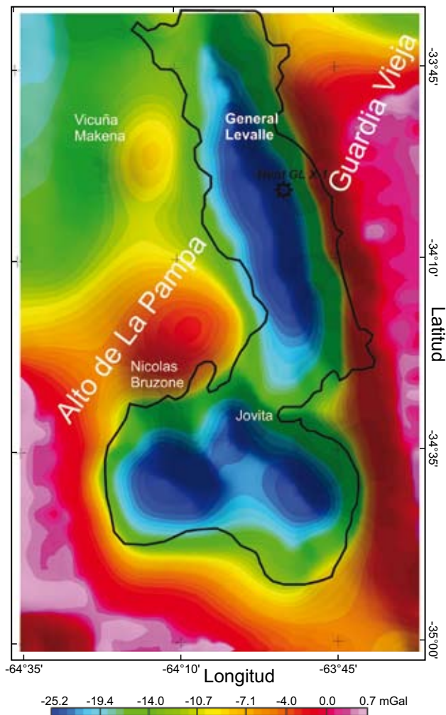
Figura 8. Carta del efecto gravimétrico de los sedimentos.
