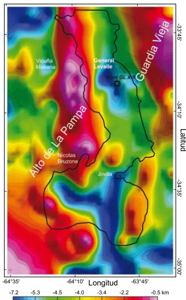
Figura 6. Mapa de basamento, obtenido por inversión gravimétrica de la anomalía residual de Bouguer.
