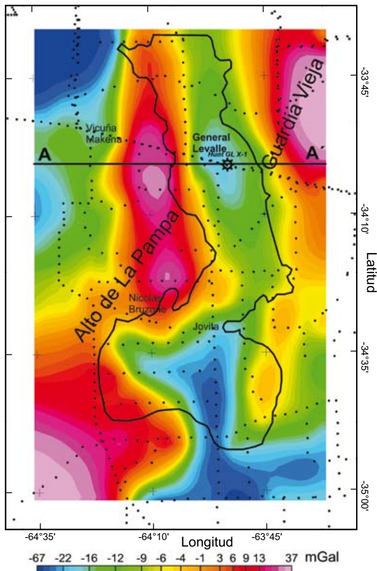
Figura 3. Mapa de anomalía de Bouguer y la distribución de puntos de gravedad medidos.
