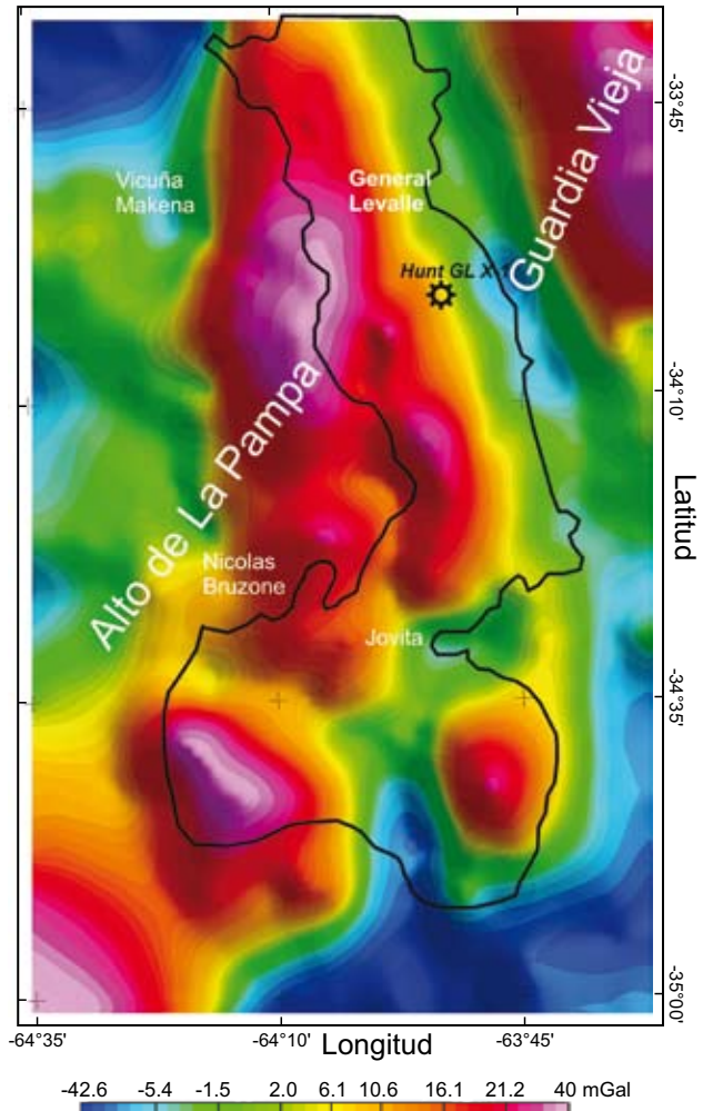
Figura 9. Mapa de anomalía de Bouguer sin el efecto gravimétrico de los sedimentos.
