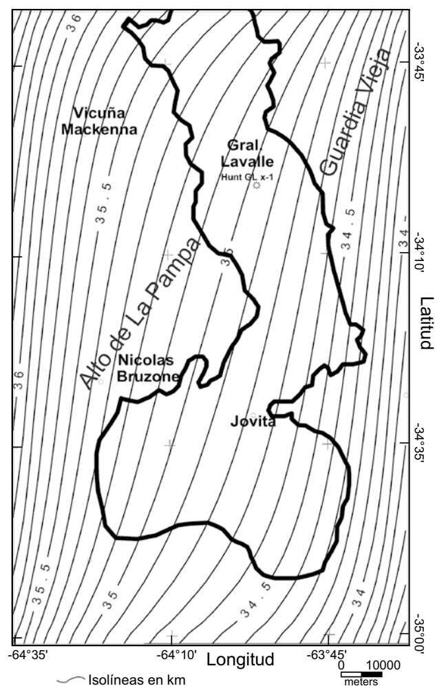
Figura 7. Superficie de la interfase corteza-manto obtenida de la inversión gravimétrica de la carta de anomalías regional de Bouguer.
