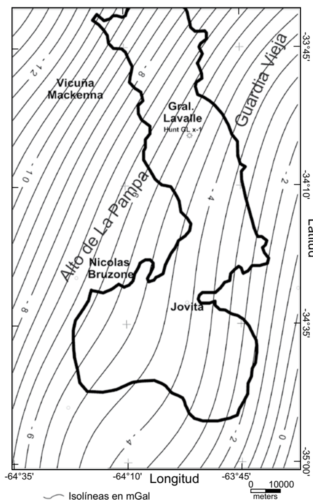
Figura 4. Mapa de anomalía regional de Bouguer.
