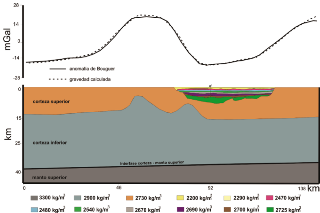
Figura 10. Modelo 2D de corteza, cuyo efecto gravimétrico justifica la anomalía de Bouguer de sección A-A' (Figura 3) a los 34° de latitud sur.
