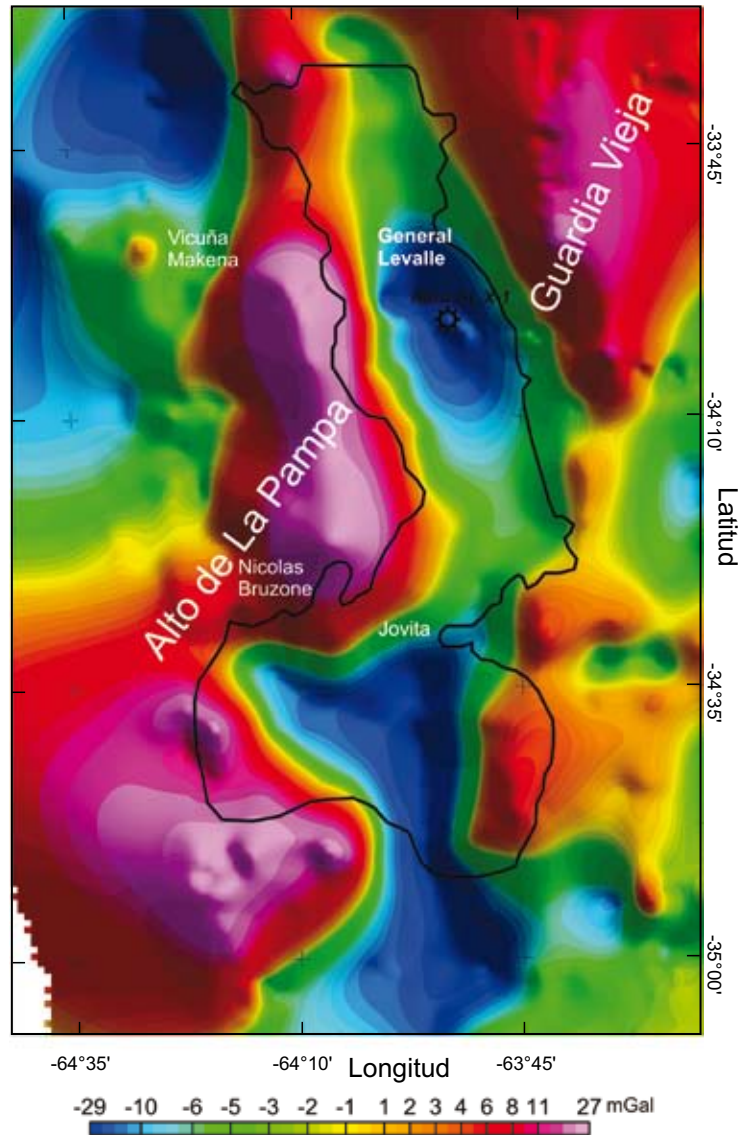
Figura 5. Carta de anomalía residual de Bouguer, obtenida mediante la prolongación ascendente a una altura de 40 km sobre el nivel del mar.
