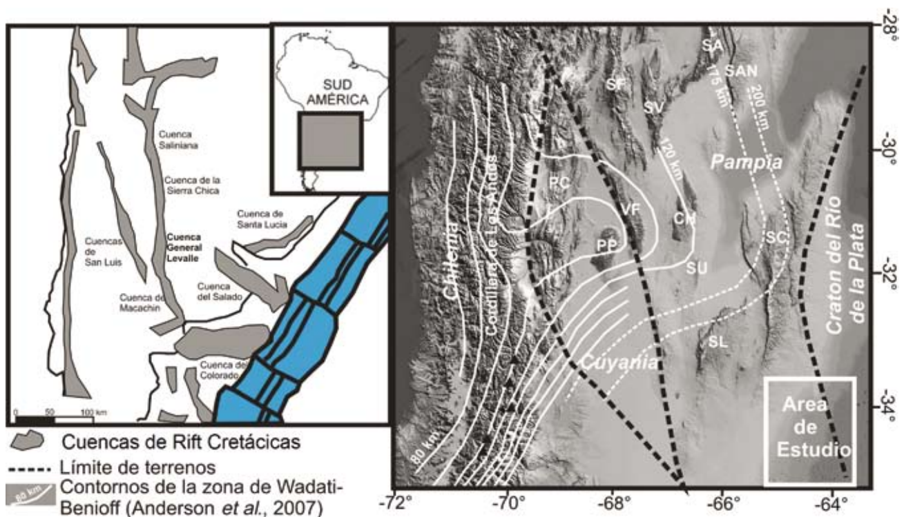
Figura 1. Ubicación geográfica del área de estudio. En la gráfica de la izquierda se indica el sistema de cuencas cretácicas. En la gráfica de la derecha, sobre el modelo de elevación digital del terreno, se graficó en blanco los contornos de la zona de Wadati-Benioff, en líneas de trazo en negro los límites de los terrenos Chilenia, Cuyanía, Pampia y Cratón del Río de La Plata. Además, se indican las principales estructuras geológicas visibles: Cordillera de Los Andes, PC: Precordillera, PP: sierra de Pie de Palo, VF: sierra de Valle Fértil, SF: Sistema de Famatina, CH: sierra de Chépes, SU: sierra de Ulapes, SL: sierra de San Luis, SV: sierra de Velasco, SA: sierra de Ambato, SAN: sierra de Ancasti y SC: sierra de Córdoba.
