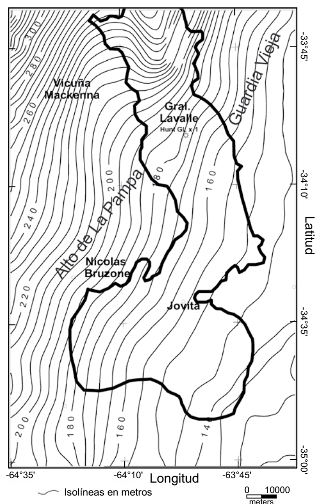
Figura 2. Modelo de elevación digital del terreno (MED), obtenido del Shuttle Radar Topography Mission (SRTM) del Servicio Geológico de Estados Unidos y la NASA. Se ha superpuesto el límite de los bordes de la cuenca General Levalle con una línea continua negra más gruesa.
