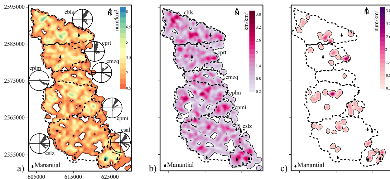
Figura 5. Mapas de densidades y diagrama de rosetas de cada una de las subcuencas. a) Densidad de alineamientos (DENNUM), b) Densidad de longitud de alineamientos (DENLON), y c) Densidad de cruzamiento de alineamientos (DENCURU).
