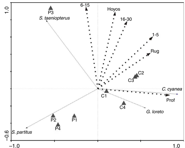
Figura 7. Gráfica del análisis de redundancia basado en las matrices de abundancias de las especies y de variables de la complejidad arrecifal durante el ciclo anual.
