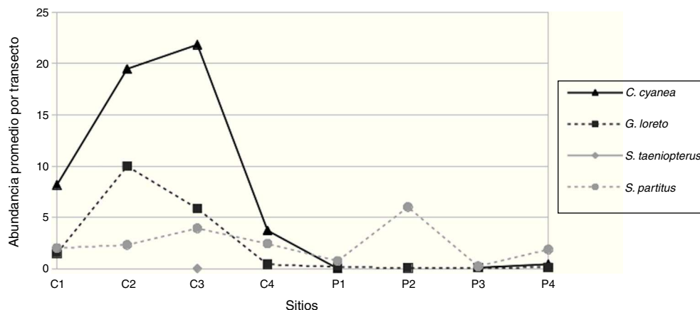
Figura 3. Abundancia promedio de cada especie en los sitios de muestreo. C: cordillera; P: parche.
