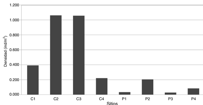
Figura 2. Densidad (ind/m 2 ) de cada especie en los sitios de muestreo. C: cordillera; P: parche.
