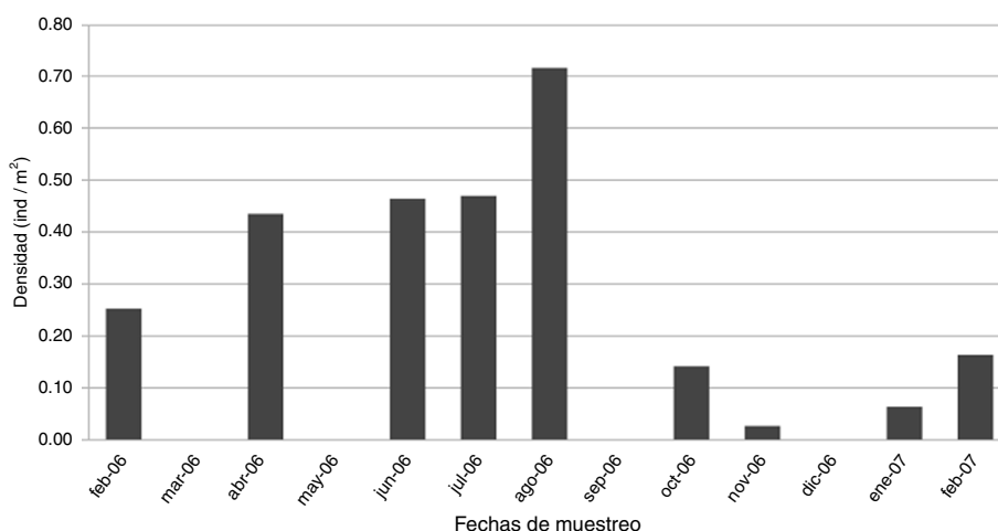
Figura 4. Densidad promedio (ind/m 2 ) para las 4 especies durante los meses de muestreo.
