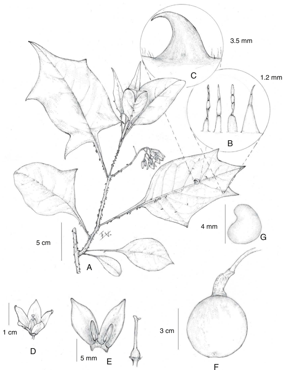
Figura 2. A, ramilla con inflorescencia; B, detalle de los tricomas del envés; C, detalle de un acúleo del envés; D, flor; E, detalle de los estambres, pétalos y pistilo; F, fruto y G, semilla (A-E con base en el holotipo y F y G con base en Cuevas, Topete y Solís, 11196).
