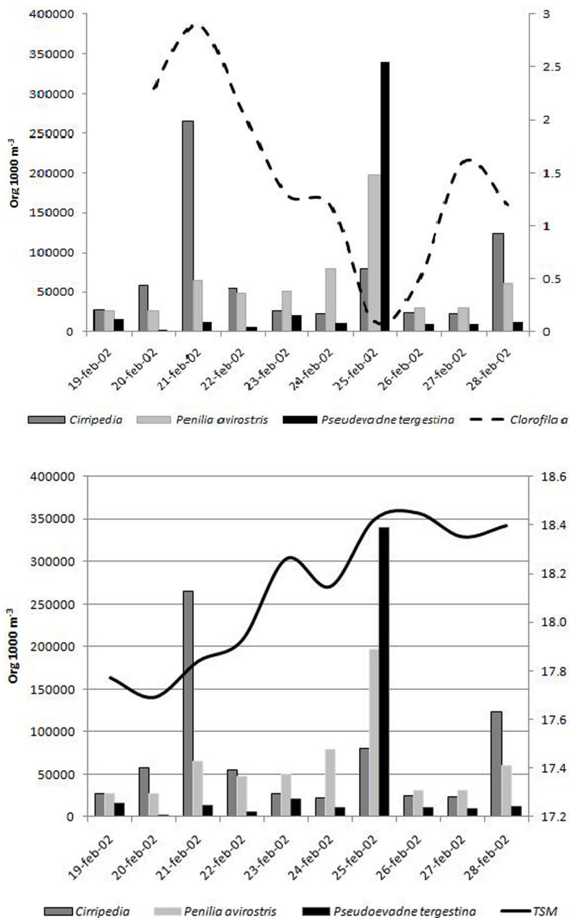
Figura 2. Variación de la densidad de nauplios de cirripedios, Penilia avirostris y Pseudevadne tergestina en la estación K2 de Bahía Magdalena, B.C.S., febrero de 2002, en relación con a), concentración de clorofila a , y b), temperatura superficial del mar.
