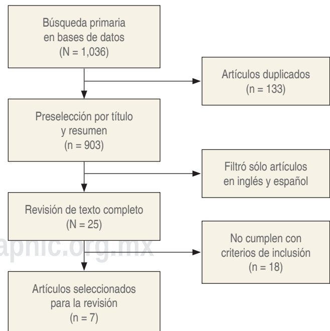
Figura 1: Flujograma PRISMA.
