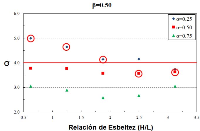
Figura 32. Factor de comportamiento sísmico Q
