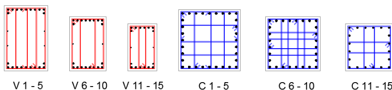
Figura 11. Armado de elementos para modelo de 15 niveles, \alpha=0.75 , \beta=0.50 , confinamiento dúctil
