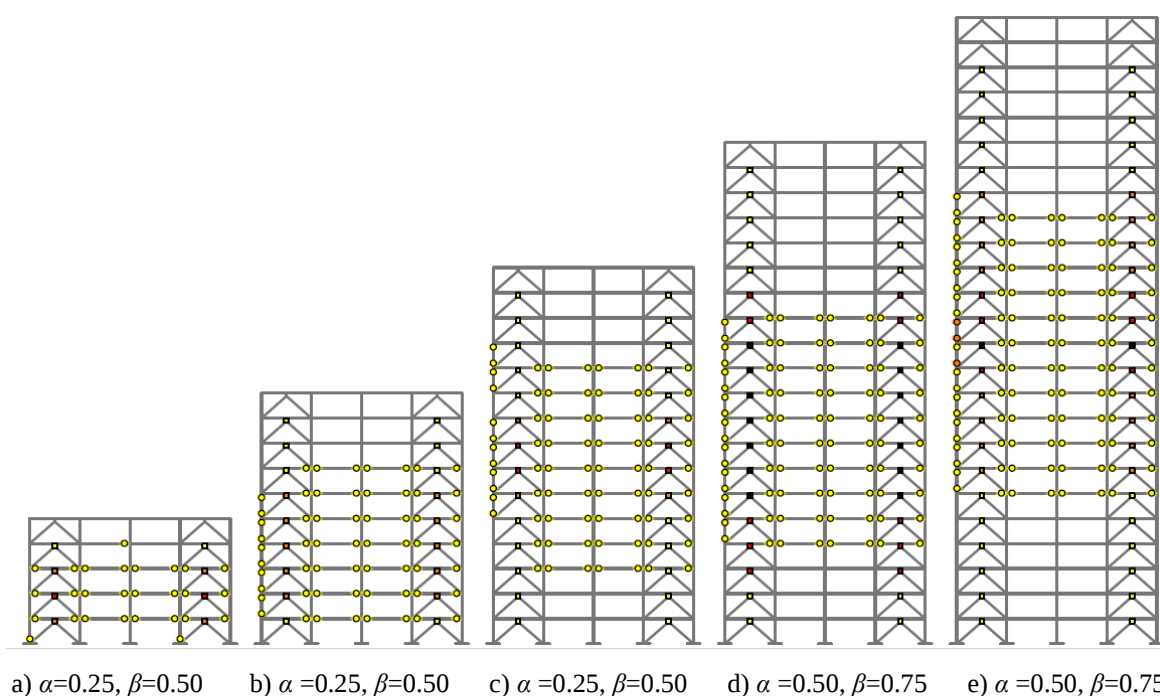
Figura 7. Mapeo de rotaciones inelásticas para balances óptimos de rigidez cuando Q \leq 4 (Tena-Colunga y Nangulasmú-Hernández 2015)
