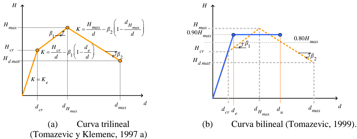
Figura 3. Idealización de la envolvente de comportamiento.
