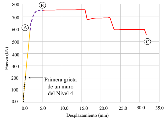
(c) Envoltura de resistencia, Nivel 1 y 4.
