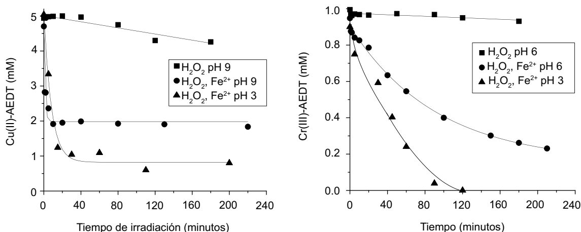
Fig. 3. Degradación de los complejos Cu(II)-AEDT y Cr(III)-AEDT mediante fotólisis en presencia de H 2 O 2 y la mezcla de H 2 O 2 y Fe 2+ en función del pH con radiación solar y una [H 2 O 2 ]:[AEDT] de 25:1
