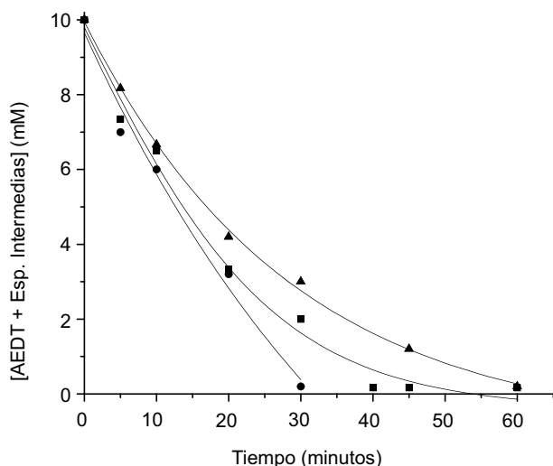
Fig. 1. Degradación del AEDT mediante el proceso foto-Fenton empleando radiación solar. 10 mM AEDT, 1 mM Fe^{2+} , pH 3. [H_2O_2]:[AEDT] de: ▲ 12.5:1, ■ 25:1, ● 37.5:1
