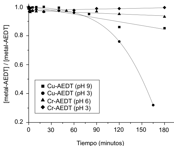
Fig. 4. Degradación de los complejos Cu(II)-AEDT y Cr(III)-AEDT con radiación solar y H 2 O 2 a diferentes valores de pH inicial con [H 2 O 2 ]:[AEDT] de 25:1
