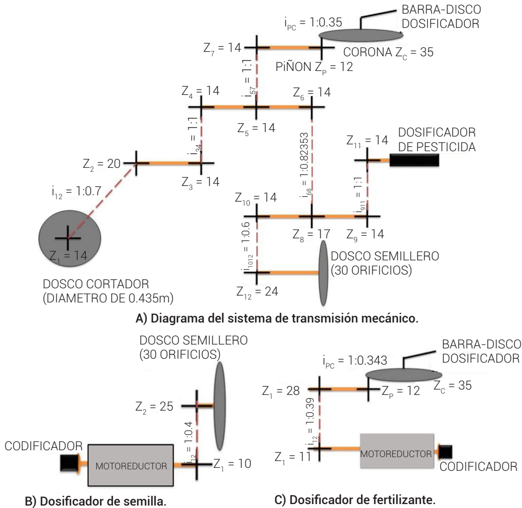
Figura 1. Diagrama del sistema de transmisión original y modificado para los dosificadores.
