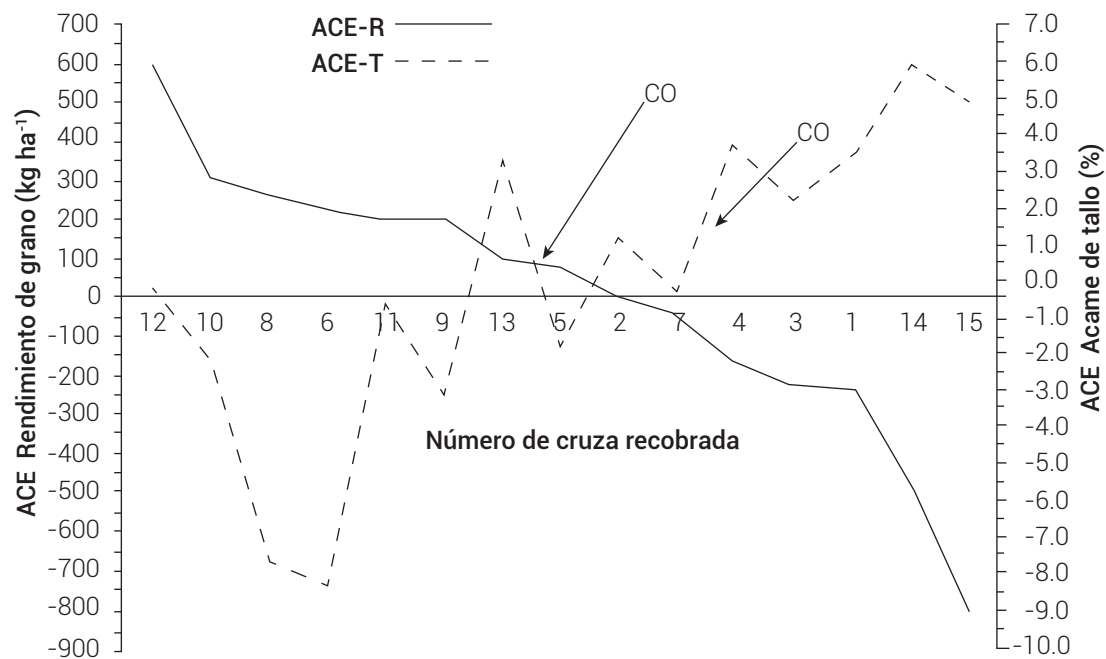
Figura 1. Aptitud combinatoria específica para rendimiento de grano (ACE-R) y porcentaje de acame de tallo (ACE-T) de cruzas recobradas formadas con sublíneas de B-3A y el probador B-4A. CO: cruce original B-3A × B-4A.
