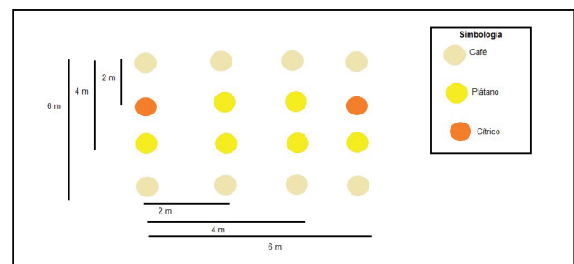
Figura 2. Diagrama de la distribución de los tres componentes del sistema agroforestal tradicional café-plátano-cítricos.
