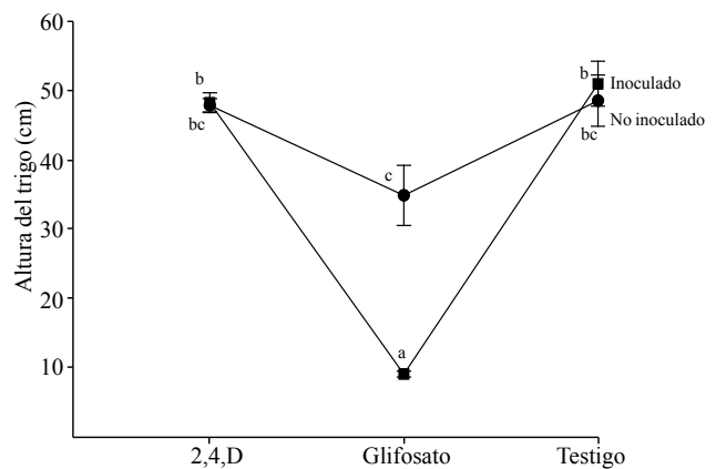
Figura 1. Efecto de dos tipos de herbicidas y la inoculación de Azospirillum en la altura del trigo var. Altiplano en invernadero. Valores con diferente letra son estadísticamente diferentes ( p \leq 0.05 ).
