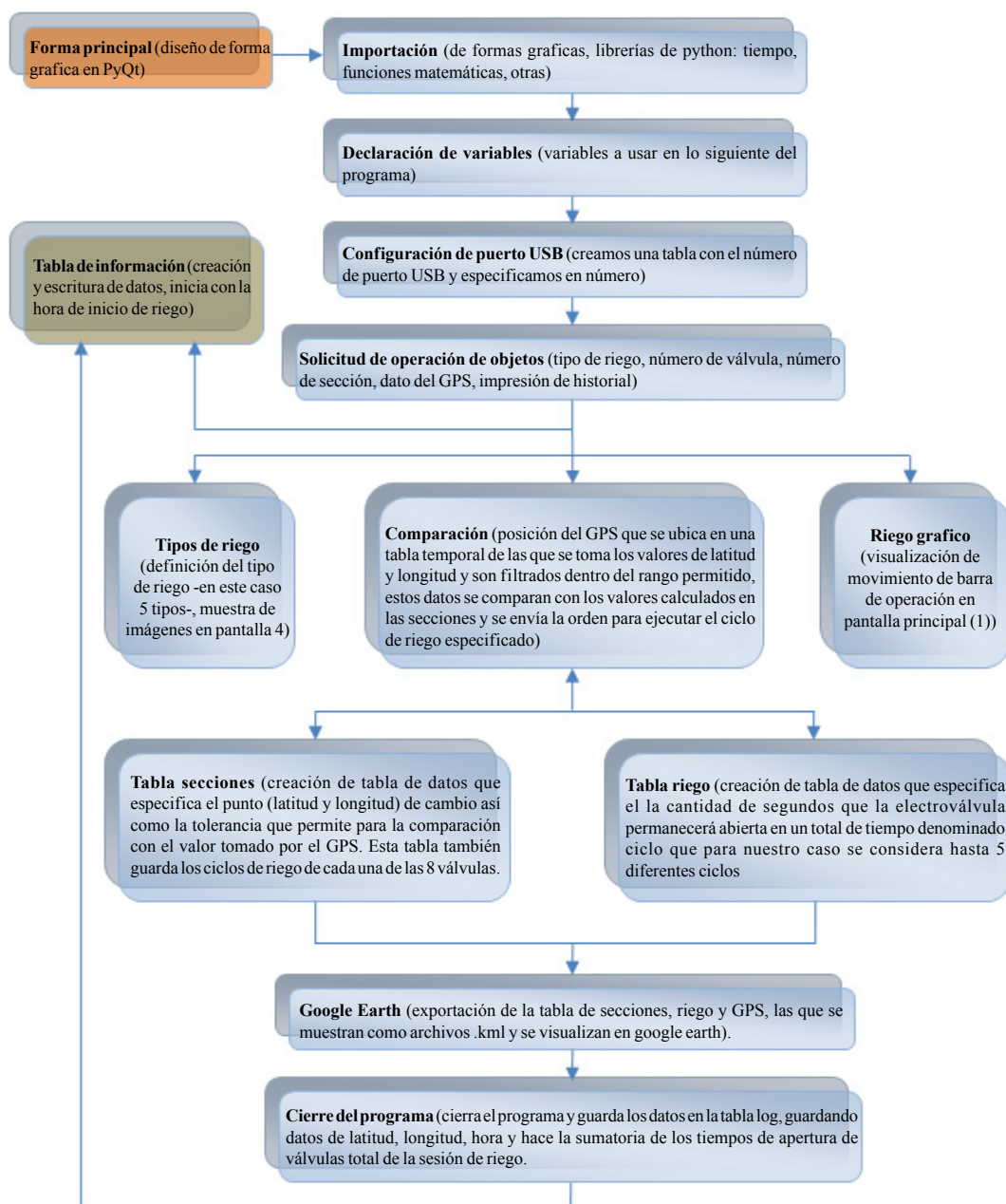
Figura 9. Diagrama de flujo del sistema de riego diferenciado.
