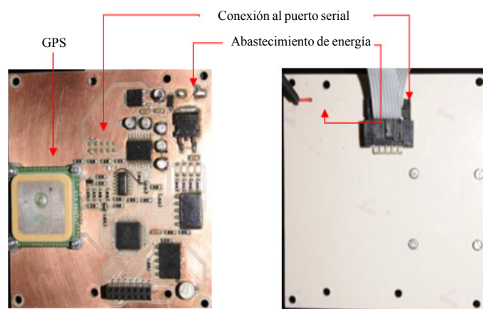
Figura 5. Diseño de la tablilla e integración de sistemas.
