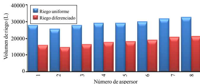
Figura 18. Comparación de riego uniforme y diferenciado en ocho aspersores del pivote central.
