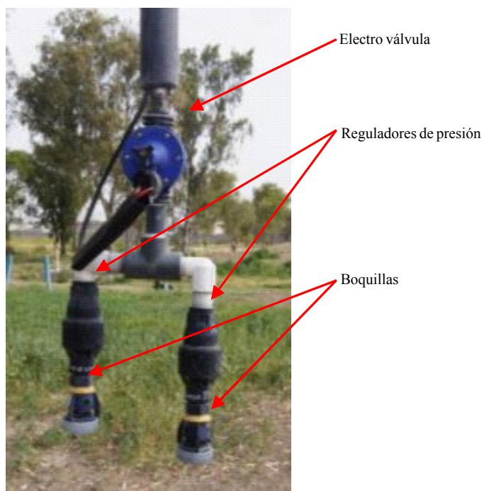
Figura 4. Ubicación de electroválvula.
