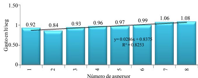
Figura 17. Gasto promedio (5 repeticiones) de últimos 8 aspersores utilizados en el riego diferenciado.
