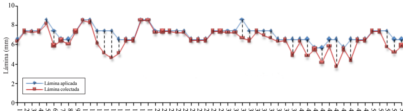
Figura 19. Comparación de la lámina aplicada con la colectada.
