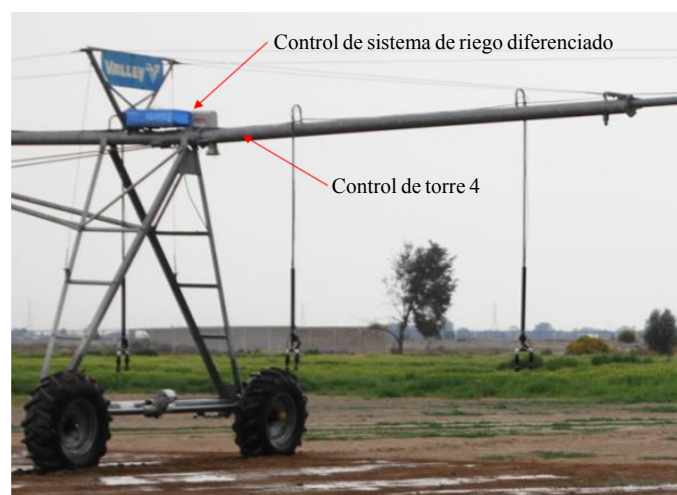
Figura 3. Ubicación del sistema de control de riego diferenciado.
