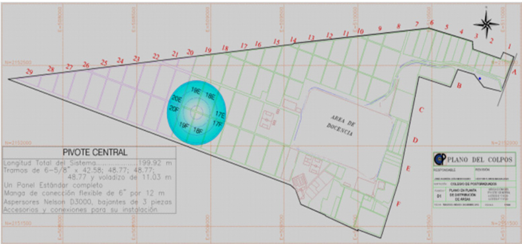
Figura 1. Plano de la ubicación del experimento en el Colegio de Postgraduados en Ciencias Agrícolas, Campus Montecillos (Ascencio, 2009).
