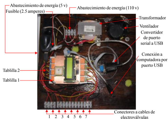
Figura 7. Diseño de la tablilla de control individualizado de las válvulas.
