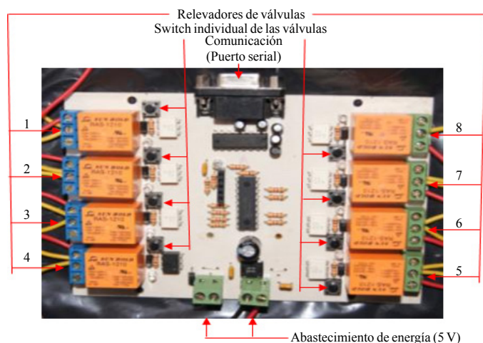
Figura 6. Diseño de la tablilla de control individualizado de las válvulas.
