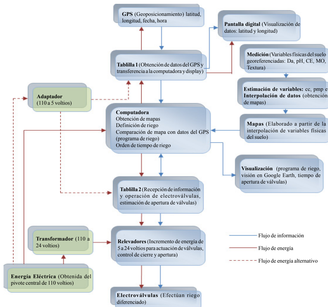
Figura 8. Diagrama de flujo de información y energía del sistema de riego diferenciado.
