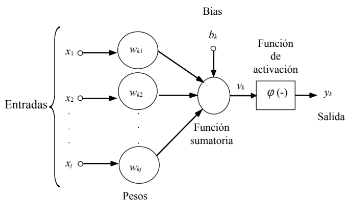
Figura 1. Esquema general de una neurona.
